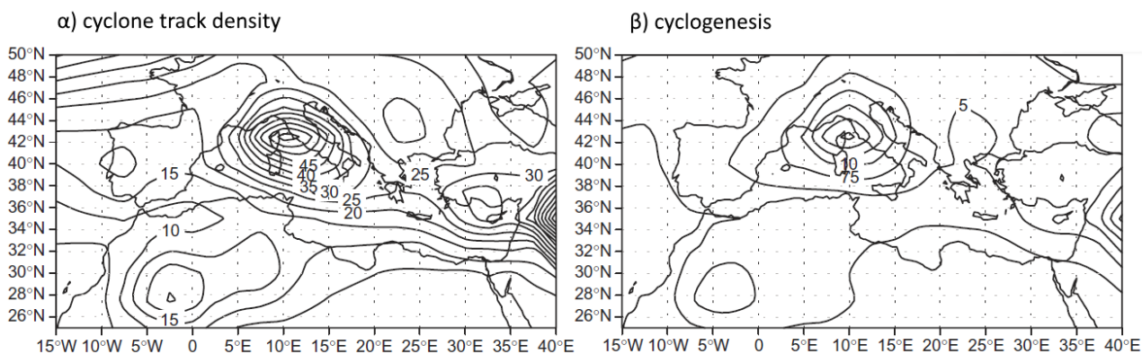
Σχήμα 2-2 α) Πυκνότητα κυκλωνικής δραστηριότητας, υπολογισμός σύμφωνα με Nissen et al. (2010), με ισοδιάσταση 5 περιστατικά/έτος/(βαθμό γεωγραφικού πλάτους) 2 β) Κυκλογένεση (περιστατικά γένεσης αναγνωρισμένων κυκλώνων) με ισοδιάσταση 2.5 περιστατικά/έτος/(βαθμό γεωγραφικού πλάτους) 2 (πηγή: Lionello 2012)
