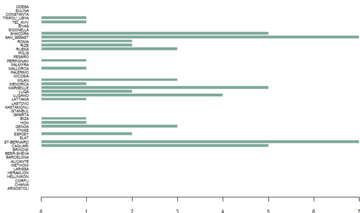
Σχήμα 4-22 Αριθμός συνδέσμων κάθε κόμβου για υστέρηση δύο ημερών και κατώτατο όριο πιθανότητας βροχόπτωσης 60%.
