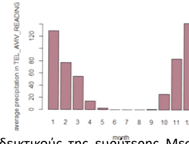
Σχήμα 3-3 Μέση τιμή μηνιαίας βροχόπτωσης για την περίοδο 1955-2001 στους σταθμούς της Ελλάδας και σε 5 ενδεικτικούς της ευρύτερης Μεσογείου.
