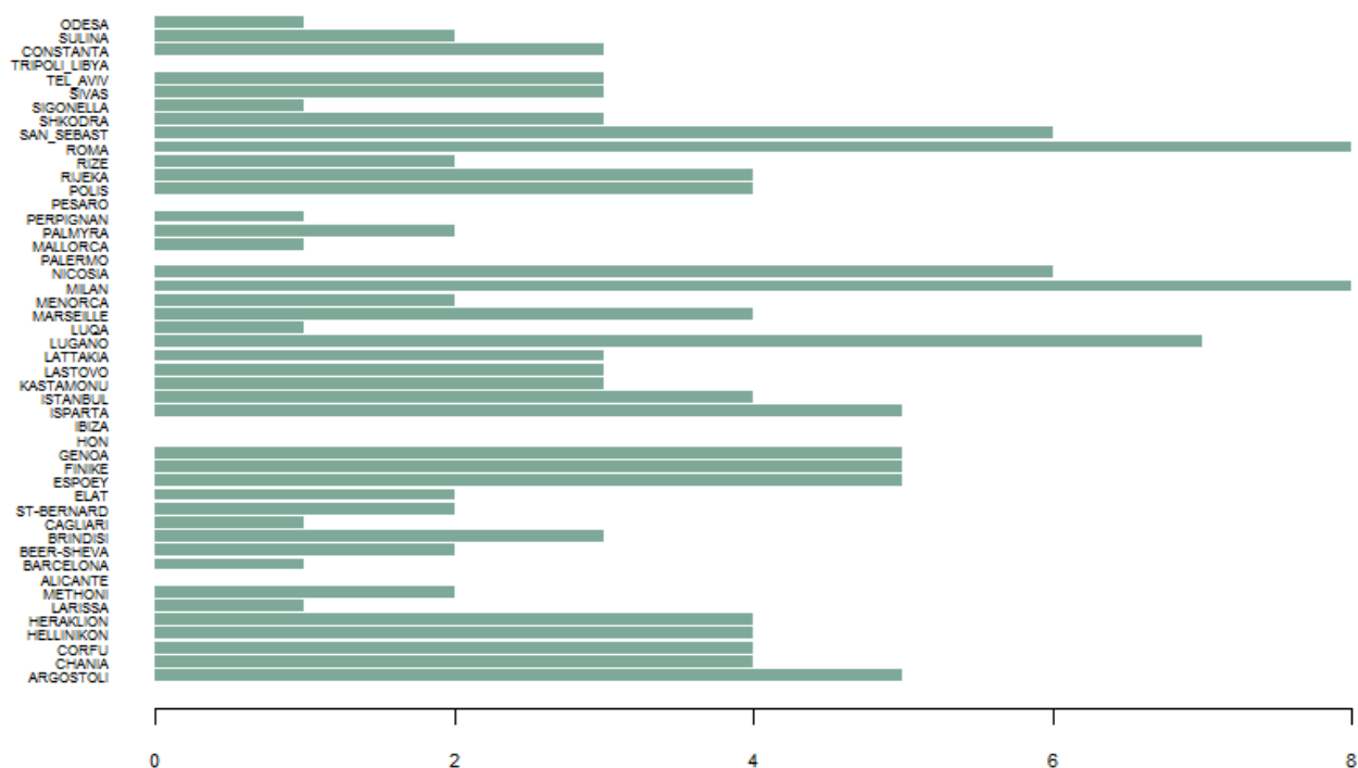
Σχήμα 4-10 Αριθμός συνδέσμων κάθε κόμβου για υστέρηση 1 και κατώτατο όριο ετεροσυσχέτισης βροχοπτώσεων 0.20.
