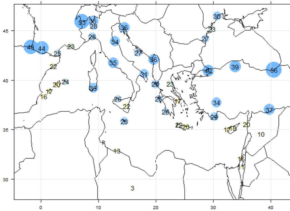
Σχήμα 4-13 Πιθανότητα βροχόπτωσης καθ' όλη τη διάρκεια του έτους.
