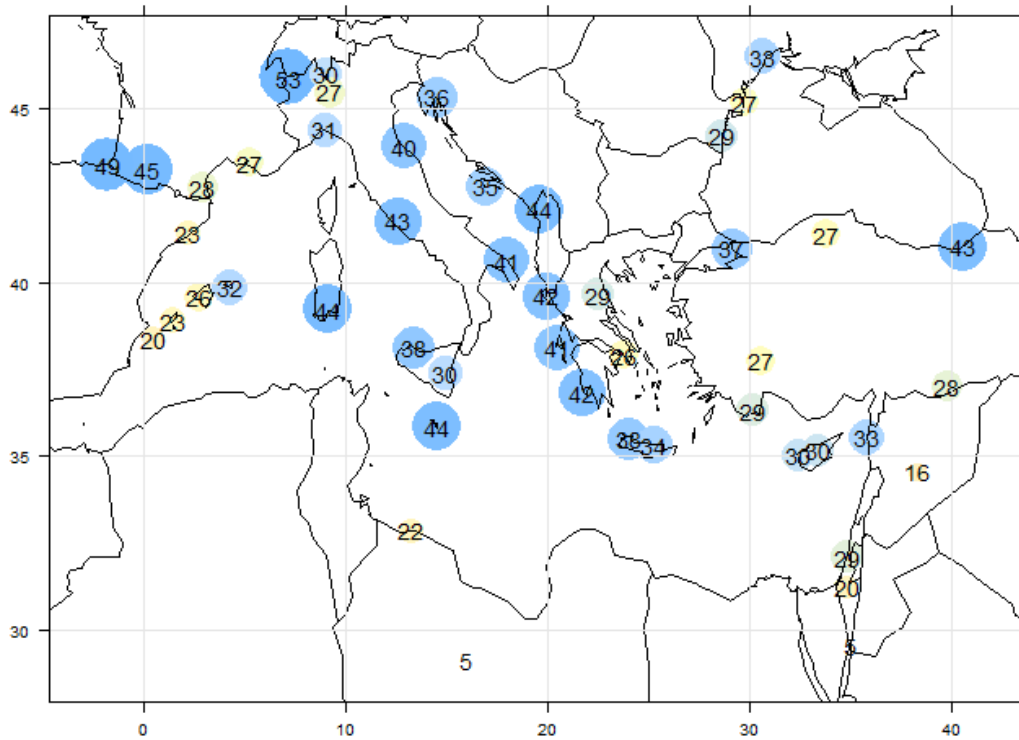
Σχήμα 4-14 Πιθανότητα βροχόπτωσης κατά την περίοδο Οκτωβρίου - Μαρτίου.
