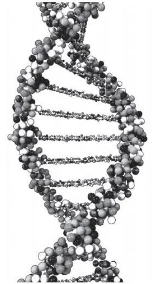
Δομή γονιδιώματος. Τρισδιάστατη απεικόνιση.
