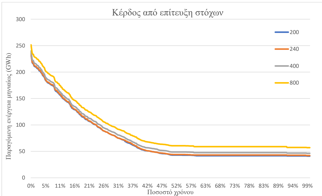
Εικόνα 6.3.3: Συνολική καμπύλη διάρκειας ενέργειας μέτρου μεγιστοποίησης κέρδους από επίτευξη στόχων σεναρίων Α1.ι
