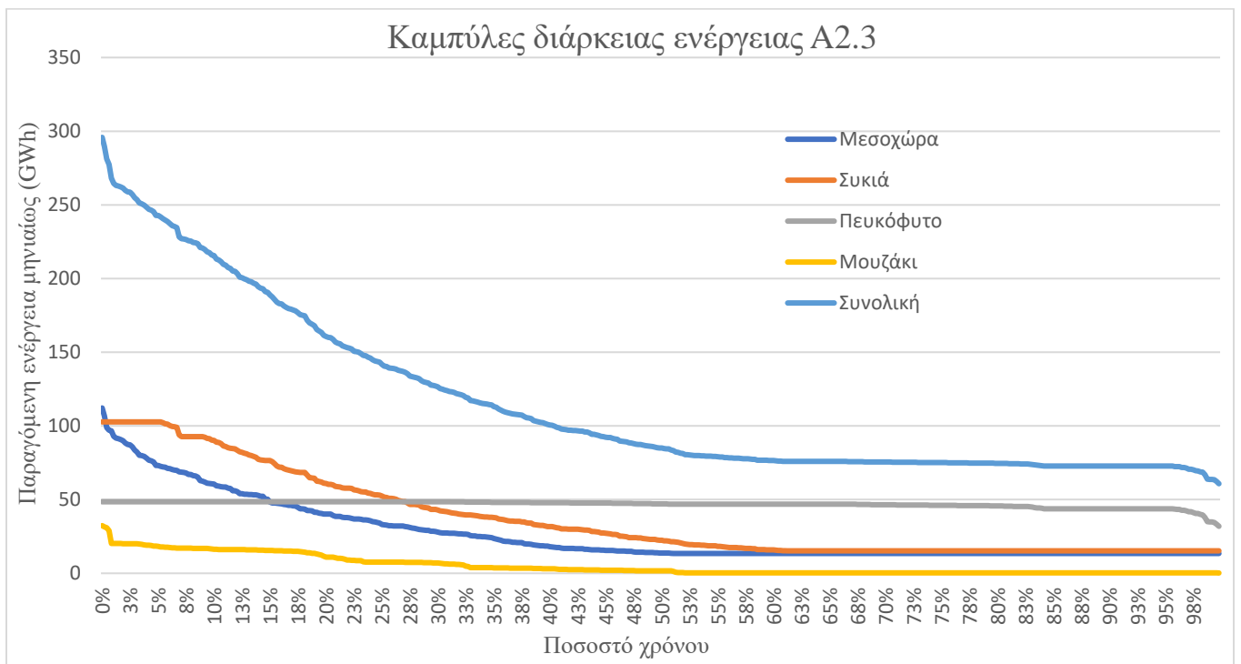
Εικόνα 6.3.8 : Καμπύλη διάρκειας ενέργειας συστήματος σεναρίου A2.3 βάσει μέτρου μεγιστοποίησης πρωτεύουσας ενέργειας
