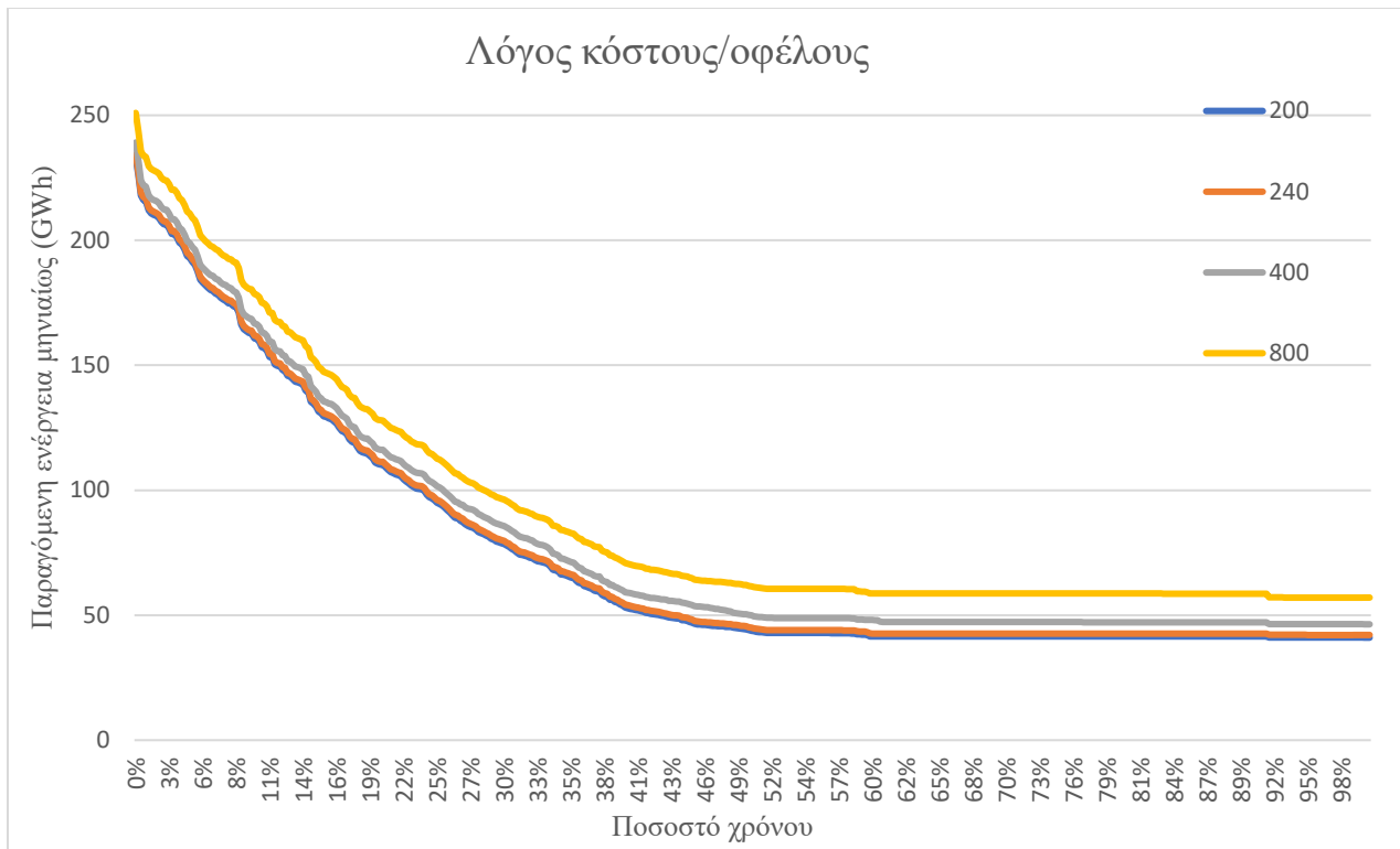
Εικόνα 6.3.2: Συνολική καμπύλη διάρκειας ενέργειας μέτρου μεγιστοποίησης λόγου κόστους/οφέλους σεναρίων Α1.ι
