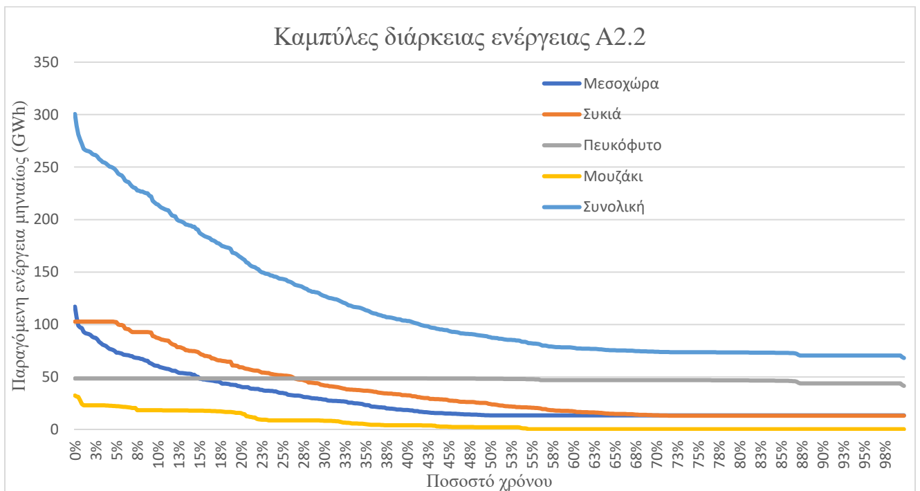
Εικόνα 6.3.6: Καμπύλη διάρκειας ενέργειας συστήματος σεναρίου A2.2 βάσει μέτρου μεγιστοποίησης προτεινόμενης ενέργειας
