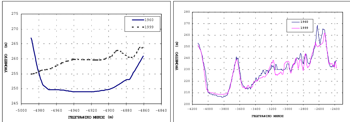
Σχήμα 3: Χαρακτηριστικές εγκάρσιες τομές του πυθμένα του ταμιευτήρα Κρεμαστών σε δύο διαφορετικές περιόδους. Figure 3: Characteristic cross sections of Kremasta reservoir's invert in two different time periods.
