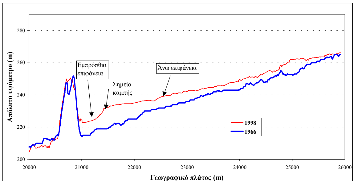
Σχήμα 4: Μηκοτομή της κοίτης του π. Αγραφιώτη στον ταμιευτήρα των Κρεμαστών. Figure 4: Longitudinal section of R. Agrafiotis at Kremasta reservoir.
