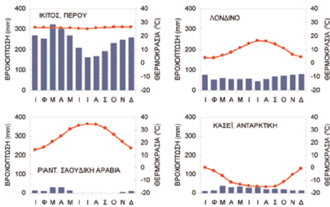
Σχ. 3. Τυπικά κλιματικά διαγράμματα που απεικονίζουν τα μέσα μεγέθη της θερμοκρασίας κάθε μήνα (κόκκινη γραμμή) και των κατακρημνισμάτων (μπλε ράβδοι) για χαρακτηριστικές κλιματικές περιοχές. Το Ικίτοζ, που βρίσκεται κοντά στον ισημερινό και παρουσιάζει σταθερά υψηλές μηνιαίες θερμοκρασίες και βροχοπτώσεις, είναι αντιπροσωπευτικό του τροπικού κλίματος. Το Λονδίνο με σταθερή βροχόπτωση σε όλους τους μήνες και μικρό θερμοκρασιακό εύρος (διαφορά θερινής και χειμερινής θερμοκρασίας) είναι χαρακτηριστικό ενός σχετικά ήπιου και υγρού κλίματος. Το Ριάντ με την ελάχιστη βροχόπτωση και τις πολύ υψηλές θερινές θερμοκρασίες είναι χαρακτηριστικό παράδειγμα ξηρού ερημικού κλίματος. Το Κάσει της Ανταρκτικής με τα πολύ μικρά κατακρημνίσματα και τις εξαιρετικά χαμηλές θερμοκρασίες είναι αντιπροσωπευτικό του πολικού κλίματος.
