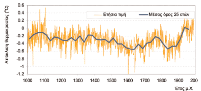
Σχ. 4. Ανακατασκευασμένο δείγμα θερμοκρασίας του Βόρειου Ημισφαιρίου (απόκλιση της μέσης ετήσιας θερμοκρασίας από τη μέση τιμή των ετών 1960-90) για την τελευταία χιλιετία με βάση συνδυασμό διάφορων υποκατάστατων δεδομένων. Πηγή δεδομένων: Jones, P. D., et al. (1998), High-resolution paleoclimatic records for the last millennium: interpretation, integration and comparison with General Circulation Model control-run temperatures. Holocene 8(4), 455–471.
