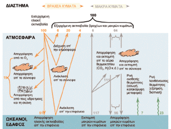
Σχ. 1. Ενεργειακό ισοζύγιο στην ατμόσφαιρα (τα μεγέθη δίνονται ως ποσοστά επί της εισερχόμενης ηλιακής ακτινοβολίας. Πηγή: Κουτσογιάννης, Δ., και Ξανθόπουλος, Θ., Τεχνική Υδρολογία , έκδοση 3η, 418 σελίδες, Εθνικό Μετσόβιο Πολυτεχνείο, Αθήνα, 1999).
