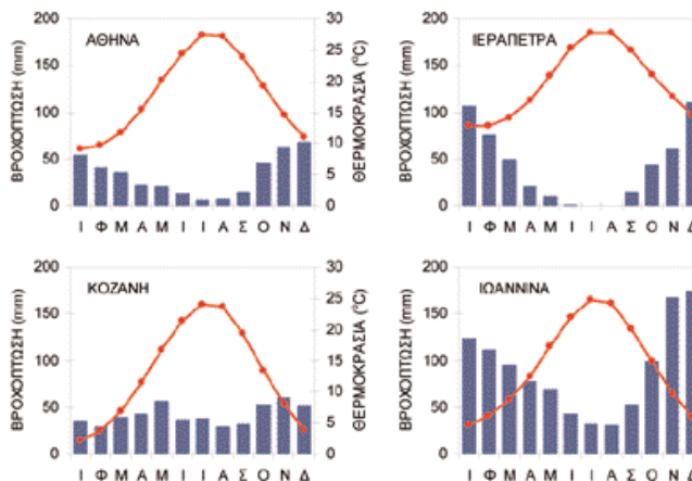
Σχ. 6. Κλιματικά διαγράμματα για πόλεις της Ελλάδας που παρουσιάζουν διαφορετικά κλιματικά χαρακτηριστικά, παρότι κατατάσσονται όλες στο ήπιο μεσογειακό κλίμα. Σε γενικές γραμμές οι θερμοκρασίες αυξάνονται προς στα νότια (Αθήνα, Ιεράπετρα), ενώ το θερμοκρασιακό εύρος (διαφορά θερινής και χειμερινής θερμοκρασίας) μεγαλώνει όσο απομακρυνόμαστε απ' τη θάλασσα (Κοζάνη, Ιωάννινα). Οι βροχοπτώσεις είναι υψηλές στη Δυτική Ελλάδα (Ιωάννινα) και πάντως μειώνονται πολύ το καλοκαίρι, με εξαίρεση όμως τους βόρειους και απομακρυσμένους απ' τη θάλασσα σταθμούς που μπορεί να εμφανίζουν σταθερή βροχόπτωση σε όλους τους μήνες (Κοζάνη).
