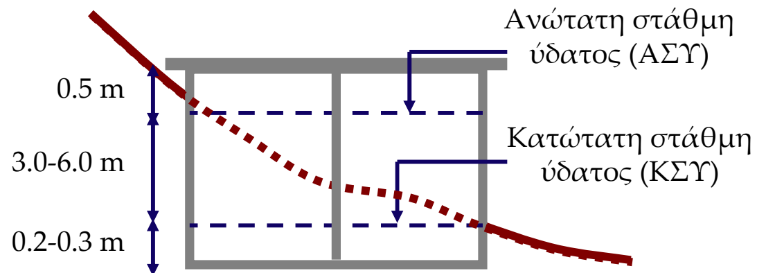
Ημιυπόγεια δεξαμενή
