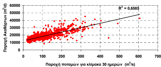
Σχήμα 5: Συσχέτιση μετρημένης παροχής ακαθάρτων –παροχής ποταμών: (πάνω) για κλίμακα ημέρας και (κάτω) για κλίμακα 30 ημερών
