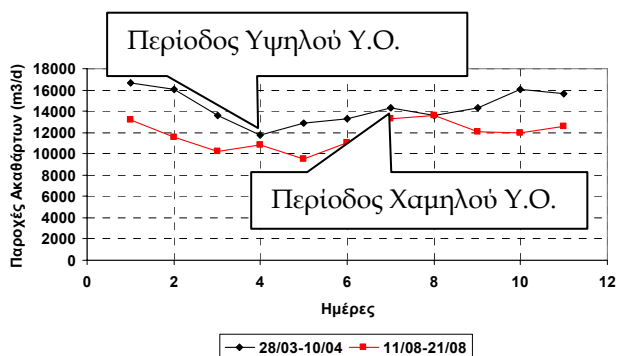
Σχήμα 3: Σύγκριση παροχής ακαθάρτων στα Ιωάννινα για ξηρές συνθήκες με υψηλή στάθμη υδροφορέα (χειμερινό δεκαήμερο) και χαμηλή στάθμη υδροφορέα (θερινό δεκαήμερο)
