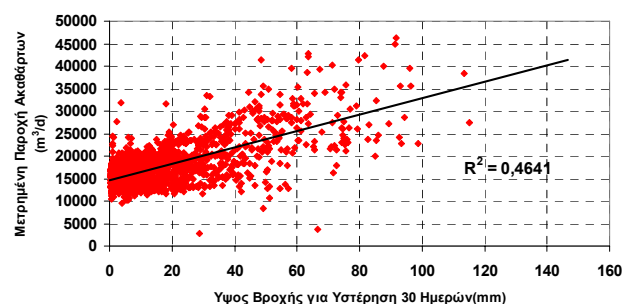
Σχήμα 4: Συσχέτιση μετρημένης παροχής ακαθάρτων – ύψους βροχής: (πάνω) για κλίμακα ημέρας και (κάτω) για κλίμακα 30 ημερών
