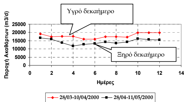
Σχήμα 2: Σύγκριση παροχής ακαθάρτων στα Ιωάννινα για βροχερές και ξηρές συνθήκες με υψηλή στάθμη υδροφορέα
