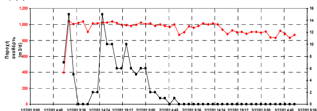
Σχήμα 10: Ωριαία διακύμανση παροχής ακαθάρτων
