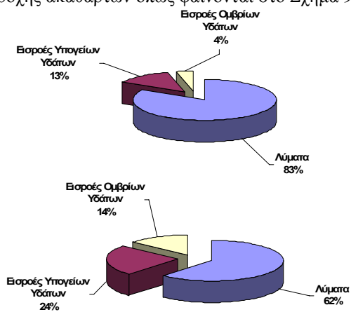
Σχήμα 9: Συνιστώσες της παροχής του δικτύου ακαθάρτων της Καρδίτσας: (πάνω) σε μέση ετήσια κλίμακα, και (κάτω) για την περίοδο που εμφανίζεται το μέγιστο 5% των τιμών της παροχής
