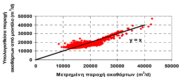
Σχήμα 6: Σχέση υπολογισθείσας – μετρημένης παροχής ακαθάρτων (Ιωάννινα)
