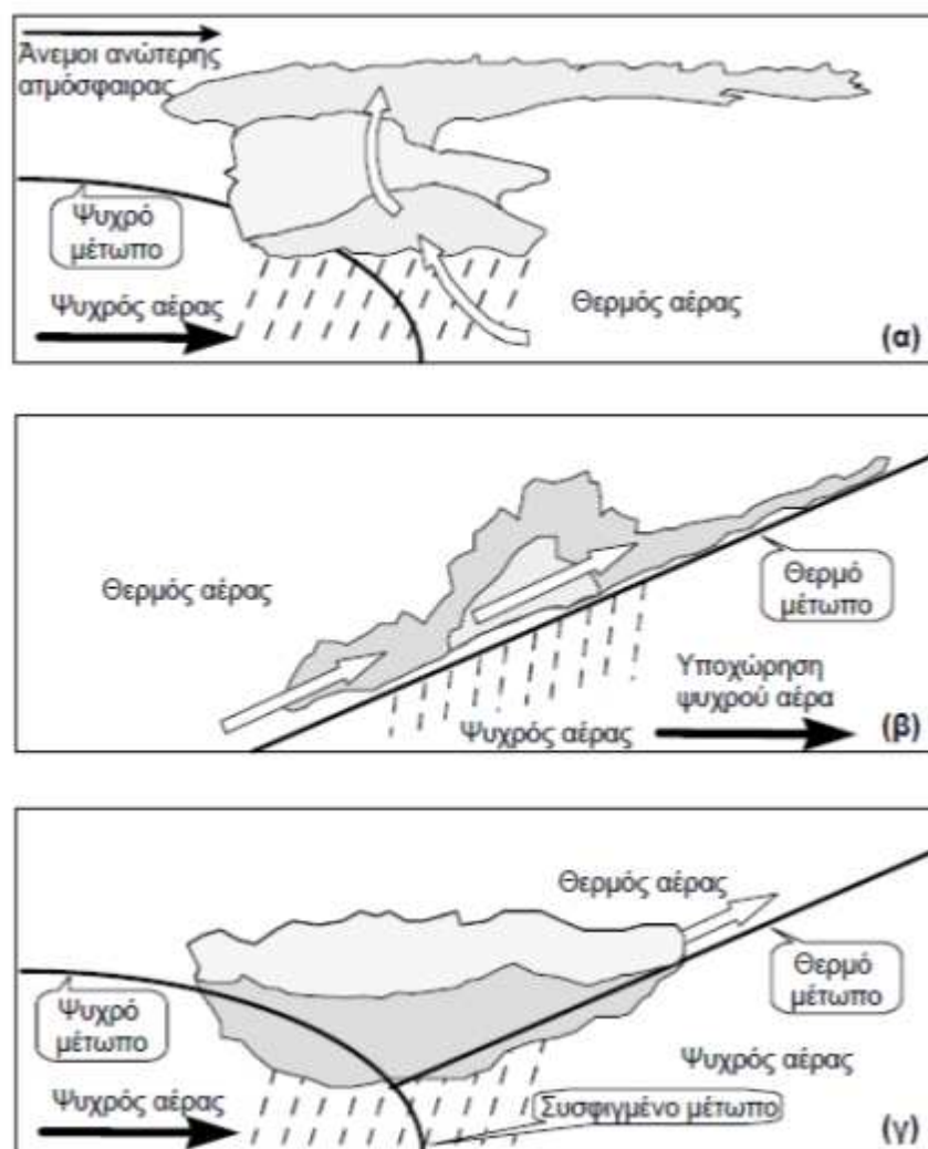
Εικόνα 0-3: Μηχανισμός Δημιουργίας Κατακρημνίσεων από Οριζόντιες Μετακινήσεις Ψυχρών και Θερμών Αέριων Μάζων (Μέτωπα). (Κουτσογιάννης & Ξανθόπουλος, Τεχνική Υδρολογία, 1999)
