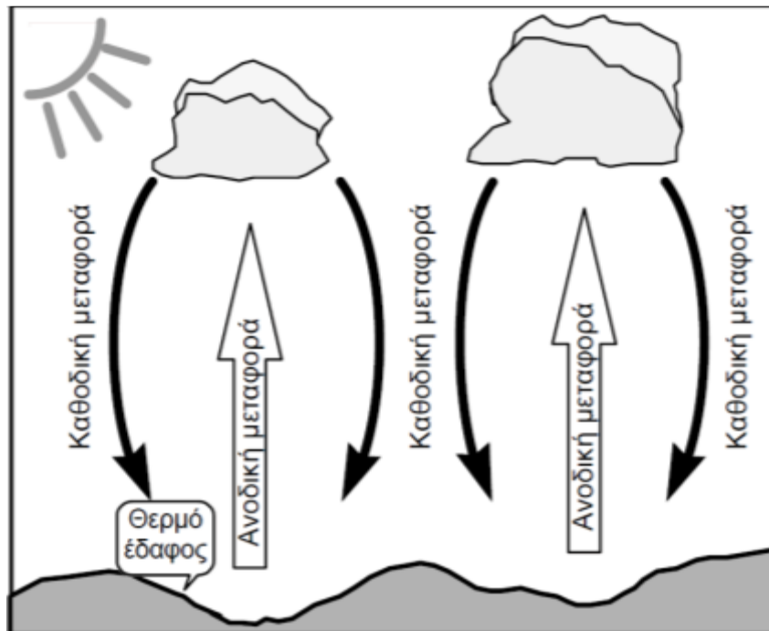
Εικόνα 0-1: Εποπτική Εικόνα Μεταγωγικού Μηχανισμού Γένεσης Βροχοπτώσεων [ (Κουτσογιάννης & Ξανθόπουλος, Τεχνική Υδρολογία, 1999)]
