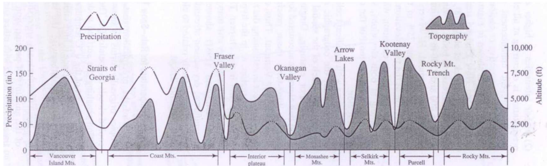
Εικόνα 0-4: Ενδεικτική Μηκοτομή της Ακτής της Βρετανικής Κολομβίας με αποτύπωση της Μέσης Τιμής της Βροχόπτωσης. (Lawrence Dingman, 1994)
