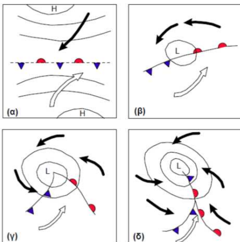
Εικόνα 0-2: Μηχανισμός Δημιουργίας Εξωτροπικών Κυκλώνων από ψυχρά (μπλε) και θερμά (κόκκινα) μέτωπα. (Κουτσογιάννης & Ξανθόπουλος, Τεχνική Υδρολογία, 1999)
