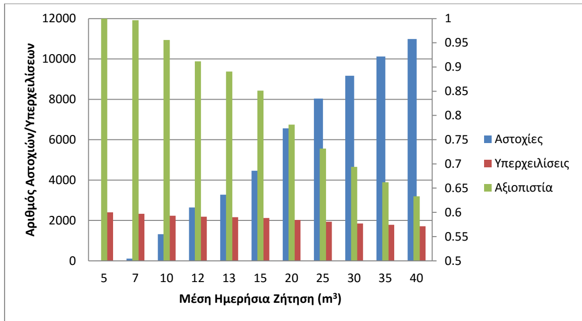
Διάγραμμα 5.6. Αριθμός αστοχιών και υπερχειλίσεων και αξιοπιστία δεξαμενής Ινώπου συναρτήσει της μέσης ημερήσιας ζήτησης σε m 3 .
