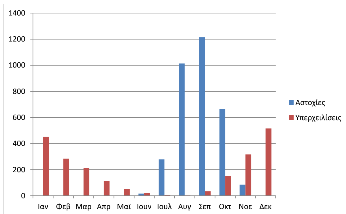
Διάγραμμα 5.7. Αριθμός αστοχιών και υπερχειλίσεων ανά μήνα, με μέση ημερήσια ζήτηση 13 m 3 , για την δεξαμενή του Ινώπου.
