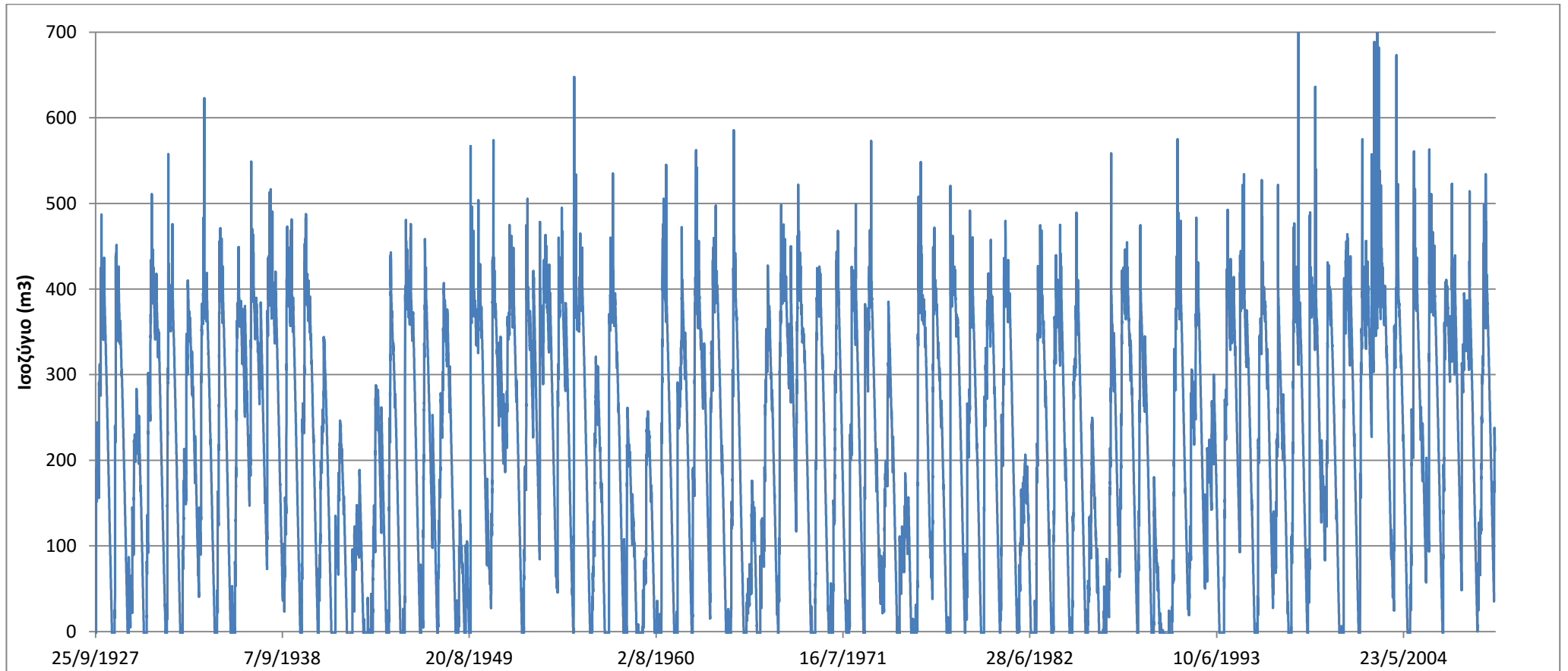
Διάγραμμα 5.3. Διακύμανση ισοζυγίου ( \text{m}^3 ) συναρτήσει του χρόνου, για την δεξαμενή του Θεάτρου, με μέση ημερήσια ζήτηση 2,25 \text{ m}^3 .
