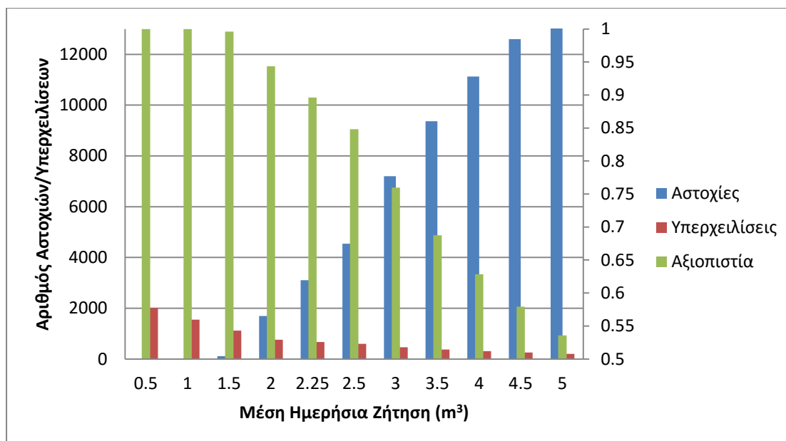
Διάγραμμα 5.1. Αριθμός αστοχιών και υπερχειλίσσεων και αξιοπιστία δεξαμενής Θεάτρου συναρτήσει της μέσης ημερήσιας ζήτησης σε m 3 .
