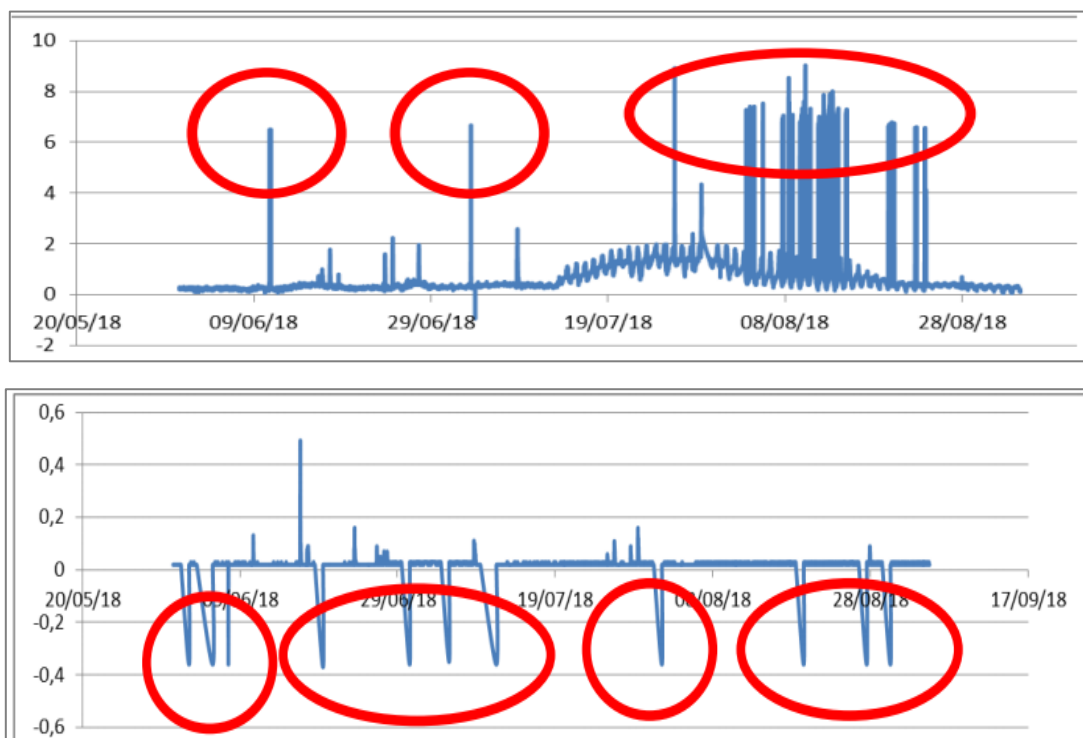
Εικόνα 5-1: Χονδροειδή σφάλματα στα πρωτογενή δεδομένα στάθμης (στιγμιαίες ακραία υψηλές τιμές-πάνω, αρνητικές τιμές – κάτω)
