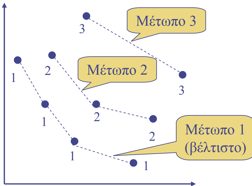
Κατάταξη σε μέτωπα κατά Goldberg (1989)
