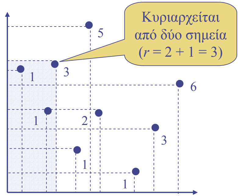
Κατάταξη κατά Fonseca and Fleming (μέθοδος MOGA, 1993)
