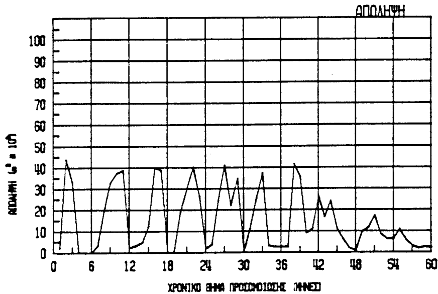
Σχ. 2 Λειτουργικά μεγέθη ταμιευτήρα Εύηνου από προσομοίωση του συστήματος Μάρνου-Εύηνου με βάση τα ιστορικά δεδομένα της περιόδου 1985-86 έως 1989-90
