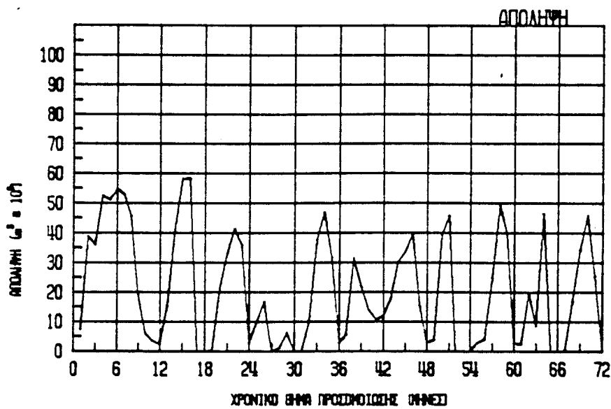
Σχ. 1 Λειτουργικά μεγέθη ταμειυτήρα Εύηνου από προσομοίωση του συστήματος Μόρνου-Εύηνου με βάση τα ιστορικά δεδομένα της περιόδου 1979-80 έως 1984-85
