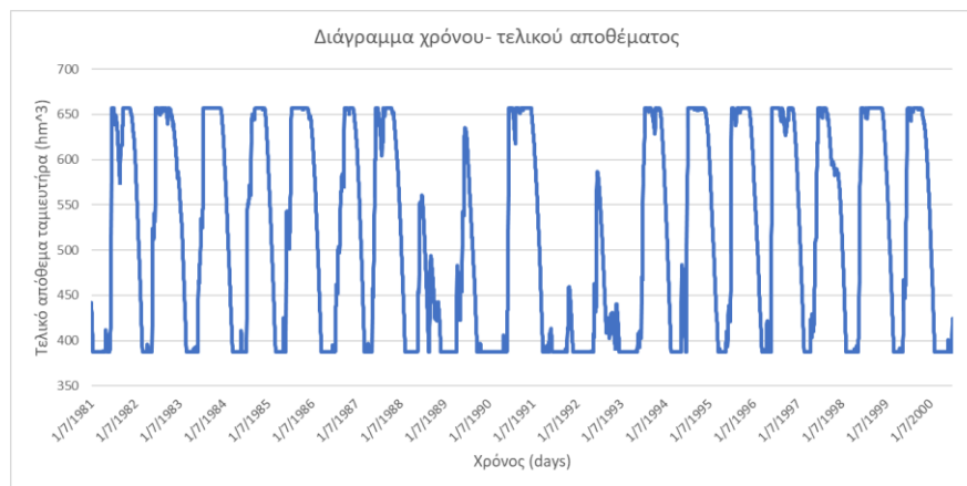
Εικόνα 6.3: Προσομοιωμένη χρονοσειράς αποθέματος ταμιευτήρα Πουρναρίου
