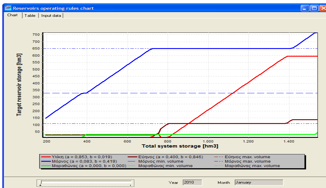
Σχήμα Β4: Γραφική παράσταση βέλτιστων κανόνων λειτουργίας ταμιευτήρων Μόρνος, Εύηνου, Υλίκης και Μαραθώνα για το στόχο μεγιστοποίησης της ασφαλούς απόδοσης του συστήματος με θεώρηση απεριόριστης παρεχόμενης υδραγωγείων και συντηρητικής χρήσης γεωτρήσεων (σενάριο Α2).
