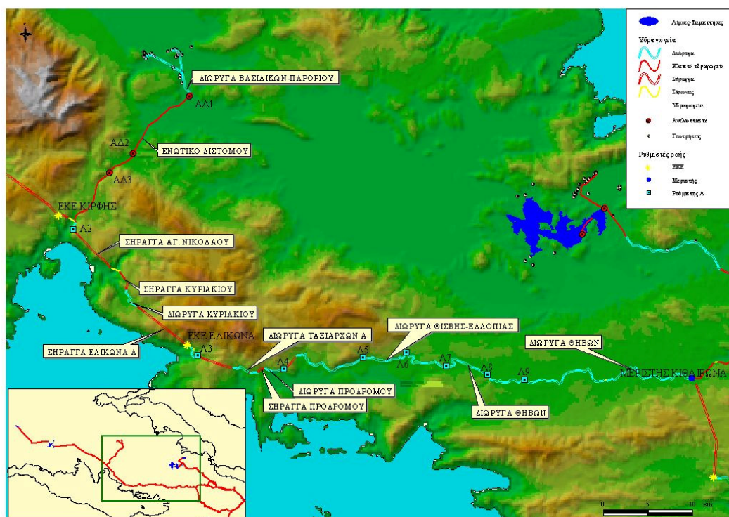
Σχήμα 4.7: Υδραγωγείο Μόρνου κατάντη ενωτικού υδραγωγείου Διστόμου
