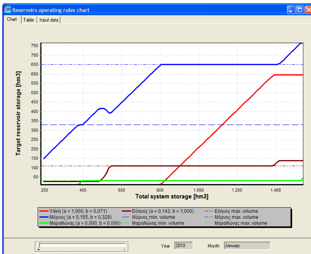
Σχήμα 5.21: Γραφική παράσταση βέλτιστων κανόνων λειτουργίας ταμιευτήρων Μόρνος, Εύηνου, Υλίκης και Μαραθώνα για το στόχο μεγιστοποίησης της ασφαλούς απόδοσης του συστήματος με θεώρηση απεριόριστης παρεχόμενης παροχότητας των υδραγωγείων και απαγόρευσης χρήσης γεωτρήσεων (σενάριο A4).
