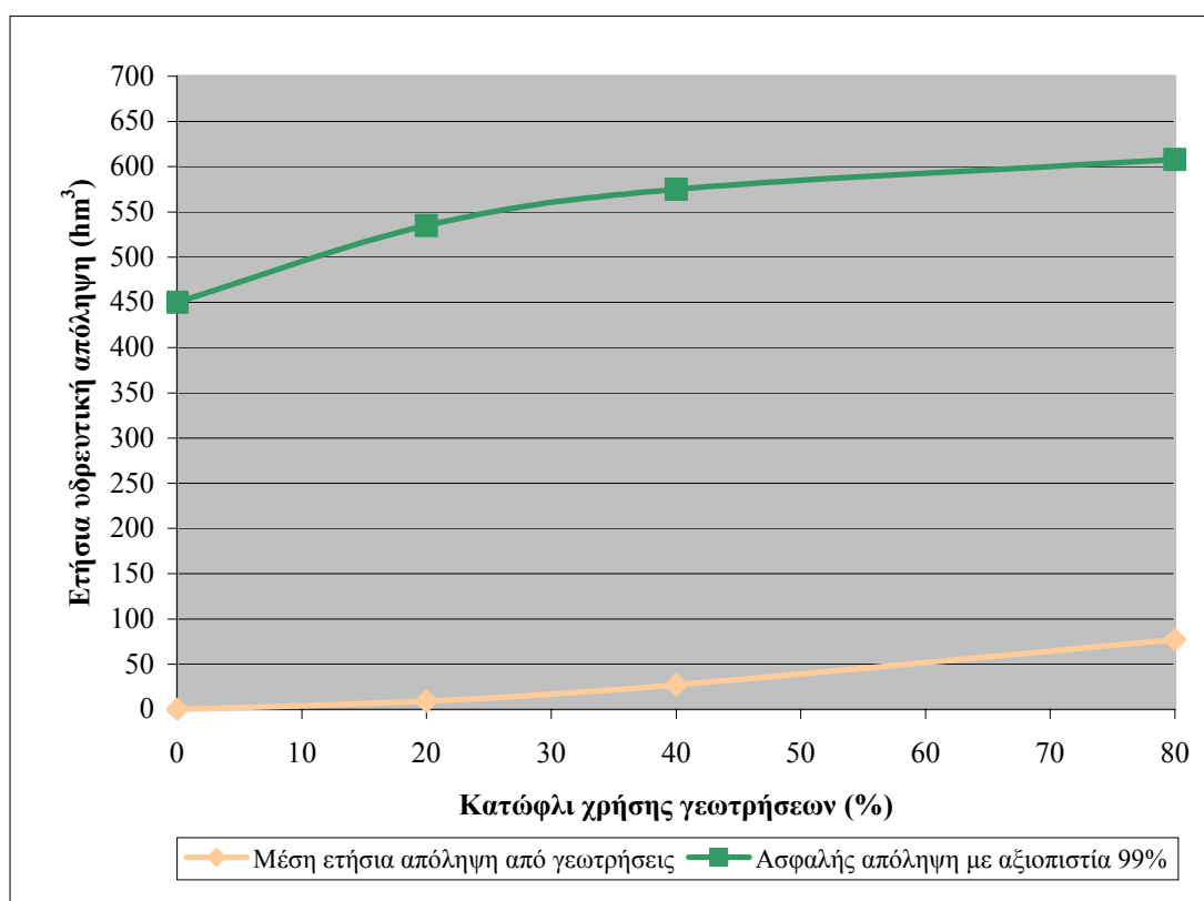
Σχήμα 5.19: Διάγραμμα της θεωρητικής ασφαλούς απόληξης του συστήματος για διάφορες πολιτικές χρήσης των γεωτρήσεων. Οι τιμές έχουν προκύψει μετά από βελτιστοποίηση των κανόνων λειτουργίας των ταμιευτήρων και με θεώρηση άπειρης παροχρητευτικότητας των υδραγωγείων.
