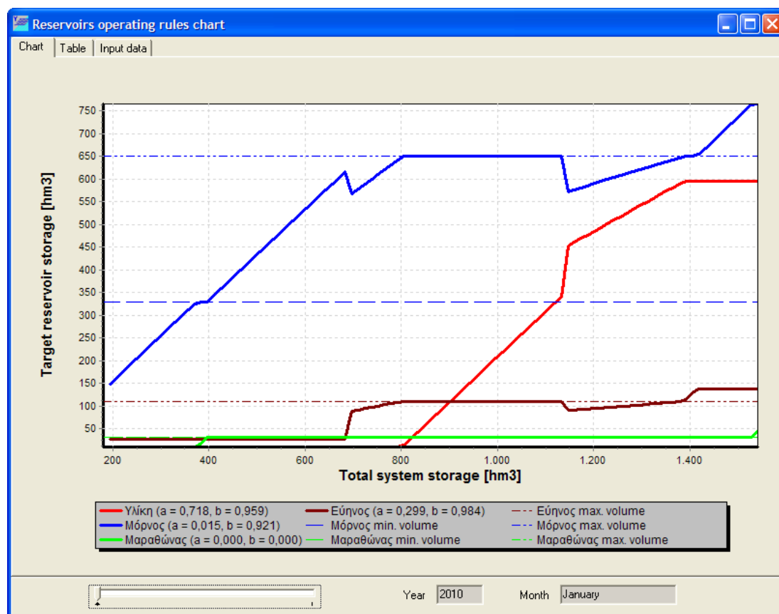
Σχήμα 5.23: Γραφική παράσταση βέλτιστων κανόνων λειτουργίας ταμιευτήρων Μόρνου, Εύηνου, Υλίκης και Μαραθώνα για το στόχο μεγιστοποίησης της ασφαλούς απόδοσης του συστήματος με θεώρηση απεριόριστης παροχευτικότητας υδραγωγείων για την επικρατούσα πολιτική χρήσης γεωτρήσεων.
