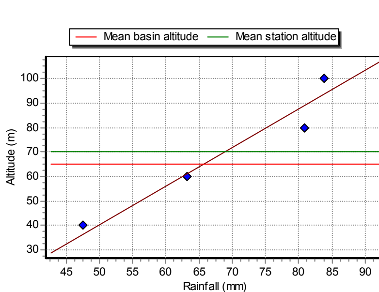
Σχήμα 8.1: Υπολογισμός βροχομετρικής βαθμίδας από τέσσερις σταθμούς.
