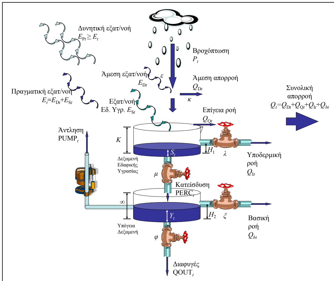
Σχήμα 8.2: Σχηματική παράσταση αδρομερούς μοντέλου βροχοπτώσης – απορροής «Ζυγός»
