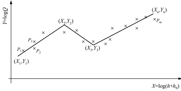
Σχήμα 5.5: Μία εν δυνάμει καμπύλη στάθμης παροχής. Τα X_i είναι δεδομένα και αναζητείται το βέλτιστο σεν Y_i
