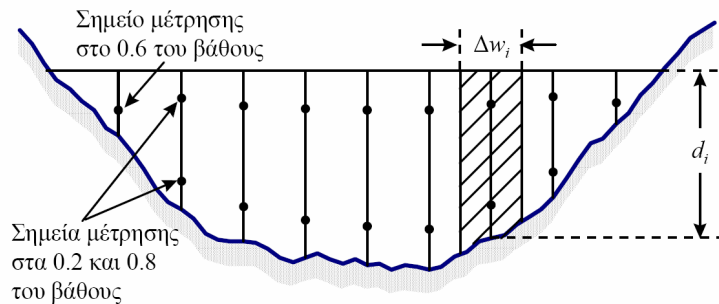
Σχήμα 5.12: Χωρισμός διατομής σε λωρίδες, υδρομετρήσεις (Κουτσογιάννης και Ξανθόπουλος, 1999, σ. 322)
