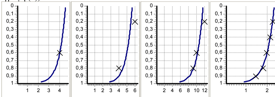
Σχήμα 5.11: Μεθοδολογίες υδρομετρήσεων: τυποποιημένες (α), (β) και (γ) στα 0.6 - 0.2 και 0.8 - 0.2, 0.6 και 0.8 του βάθους. 5 τυχαία σημεία (δ) λογαριθμική καμπύλη με βέλτιστη προσαρμογή σε 5 τυχαία σημεία.
