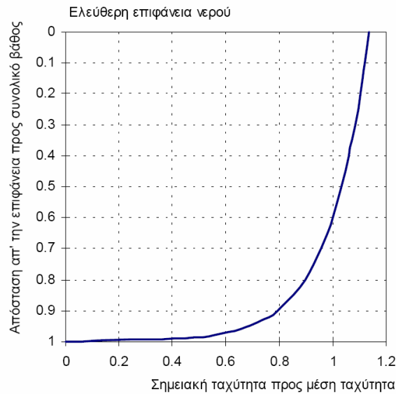
Σχήμα 5.13: Τυπική διανομή ταχυτήτων σε μια κατακόρυφη διατομή υδατορεύματος (Κουτσογιάννης & Ξανθόπουλος, 1999, σ. 321)
