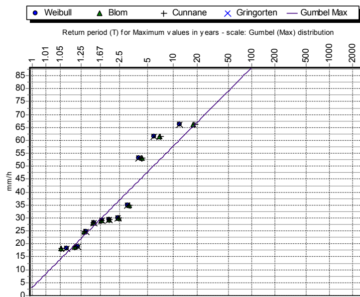
Σχήμα 9.1: Εμπειρικές κατανομές Weibull, Blom, Cunnane, Gringorten. Ετήσια μέγιστα έντασης ωριαίων βροχοπτώσεων. Σταθμός «Πολυτεχνειούπολης» 1993-4 – 2003-4
