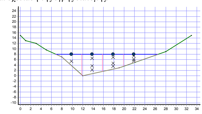
Σχήμα 5.10: Συνεδρία υδρομέτρησης όπως εμφανίζεται στην εφαρμογή του Υδρογνώμονα. Με πράσινο χρώμα η διατομή, με μπλε η υγρή διατομή, θέσεις στήλης υδρομετρήσεων (τελείες), λωρίδες (ροζ) και υδρομετρήσεις (X).
