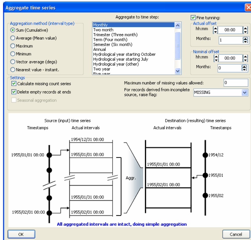
Σχήμα 4.2: Οθόνη ρύθμισης των παραμέτρων της συνάθροισης.
