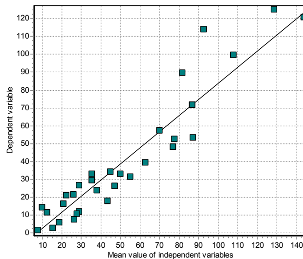
Σχήμα 7.2: Διάγραμμα διασποράς πολλαπλής γραμμικής παλινδρόμησης για την βροχόπτωση μηνός Απριλίου. Εξαρτημένη μεταβλητή: σταθμός Αλιάρτου, ανεξάρτητες μεταβλητές: σταθμοί Αμφισσας, Αταλάντης, Αγ. Τριάδας ( \delta=0.90 ).
