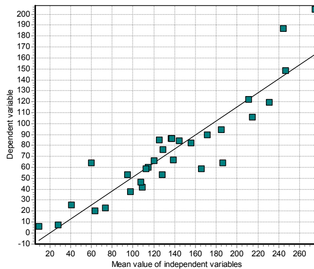
Σχήμα 7.1: Διάγραμμα διασποράς απλής γραμμικής παλινδρόμησης μηνός Φεβρουαρίου για την βροχόπτωση στους σταθμούς Αλιάρτος, Αγ. Τριάδα ( \delta=0.83 ).
