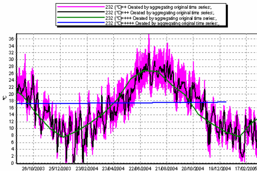
Σχήμα 4.3: Συνάθροιση ωριαίας χρονοσειράς μέσω τιμών θερμοκρασίας σε ημερήσια, μηνιαία και ετήσια χρονοσειρά μέσω τιμών. Σταθμός Πολυτεχνειούπολης Ζωγράφου.
