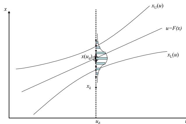
Σχήμα 9.7: Όρια εμπιστοσύνης x_U , x_L , πειράματα x_k και κατανομή τους περί του σημείου x(u_d) .
