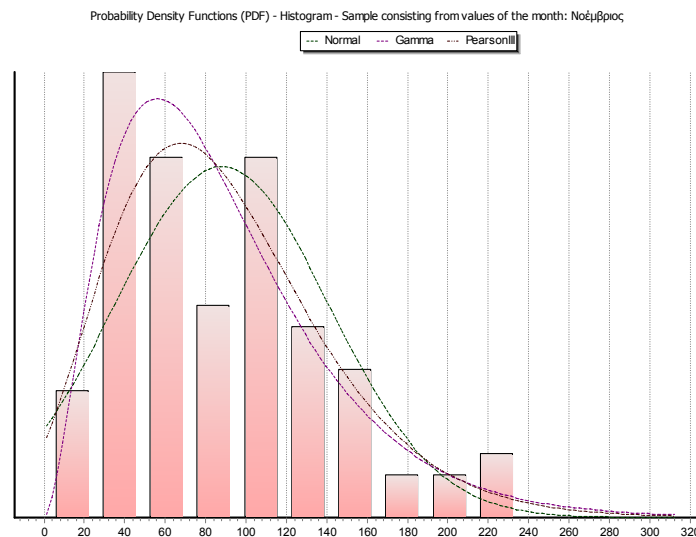
Σχήμα 9.6: Ιστόγραμμα και Σ.Π.Π. Κανονικής κατανομής, κατανομής Γάμα και Pearson-III, στο δείγμα μηνιαίων τιμών Νοεμβρίου στον σταθμό του Αλιάρτου.
