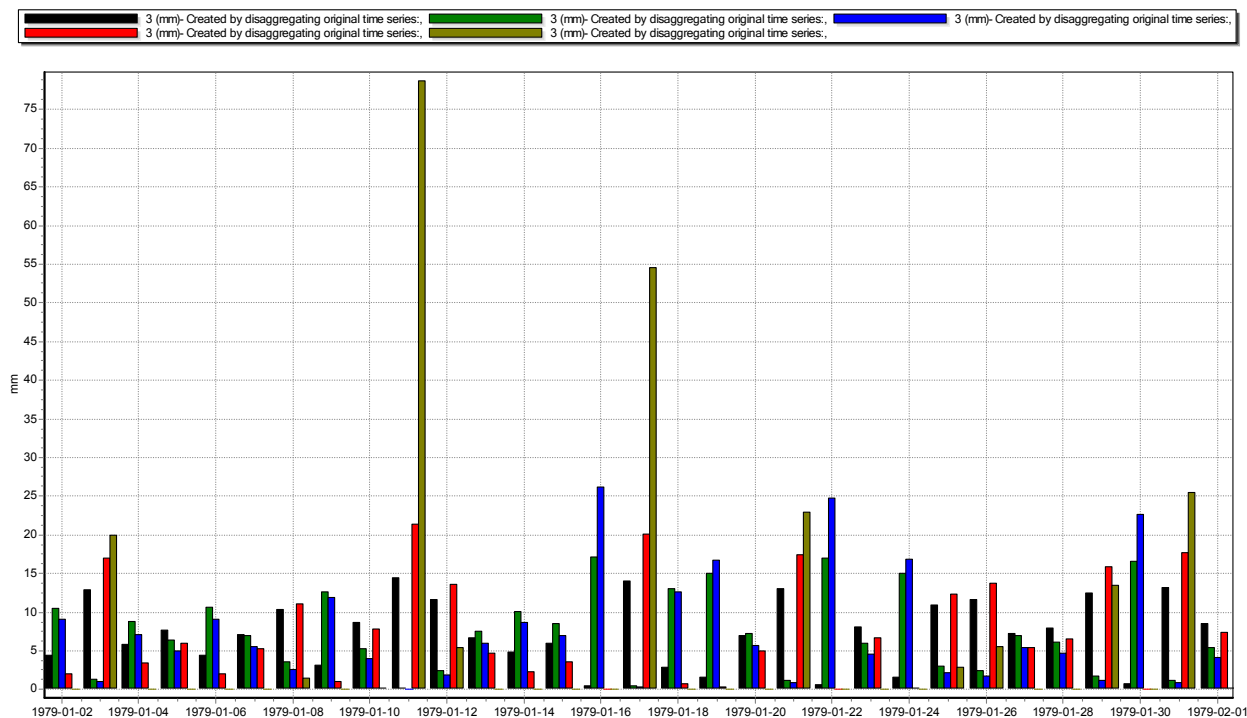
Σχήμα 4.4: Σύγκριση των τυχαίων μοντέλων, επιμερισμός της μηνιαίας τιμής Ιανουαρίου σε 31 τυχαίες τιμές. Από αριστερά προς δεξιά: Ομοιόμορφη κατανομή, εκθετικό, λογαριθμικό, τετραγωνικό και ανώτερης τάξης μοντέλο.
