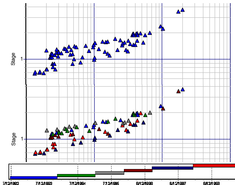
Σχήμα 5.4: Διαχωρισμός των υδρομετρήσεων σε ομοιογενείς περιόδους (με διαφορετικό χρωματισμό). Υδρομετρήσεις 1992-1998 από τον σταθμό «Πόρος Ρηγανίου» στον ποταμό Εύηνο.
