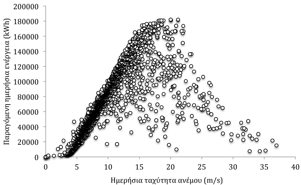
Σχήμα 6.3 Η ημερήσια παραγόμενη ενέργεια της ανεμογεννήτριας συναρτίζεται της ημερήσιας ταχύτητας ανέμου με χρήση των μέσων ωριαίων ταχυτήτων ανέμου
