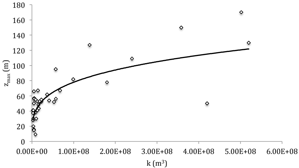
Σχήμα 8.2 Η συνεχής καμπύλη αντιστοιχεί στη z_{\max}=0.533*k^{0.27} . Με \diamond συμβολίζεται η συσχέτιση z_{\max} - k των ταμιευτήρων που χρησιμοποιήθηκαν.
