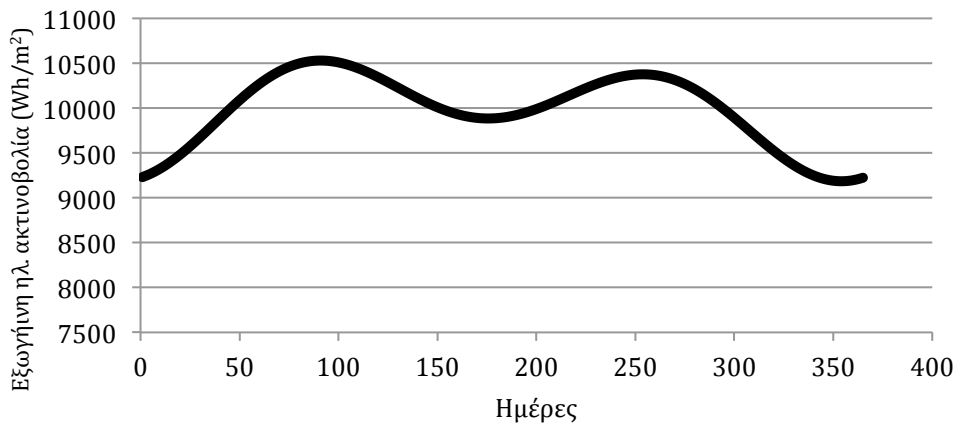
Σχήμα Δ.4 Ημερήσια εξωγήινη ηλιακή ακτινοβολία σε επίπεδο με κλίση 32°.
