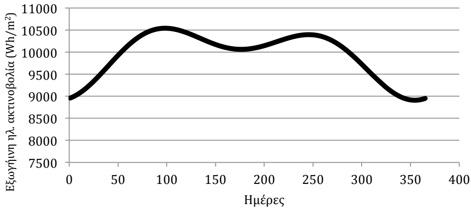
Σχήμα Δ.3 Ημερήσια εξωγήινη ηλιακή ακτινοβολία σε επίπεδο με κλίση 30°.
