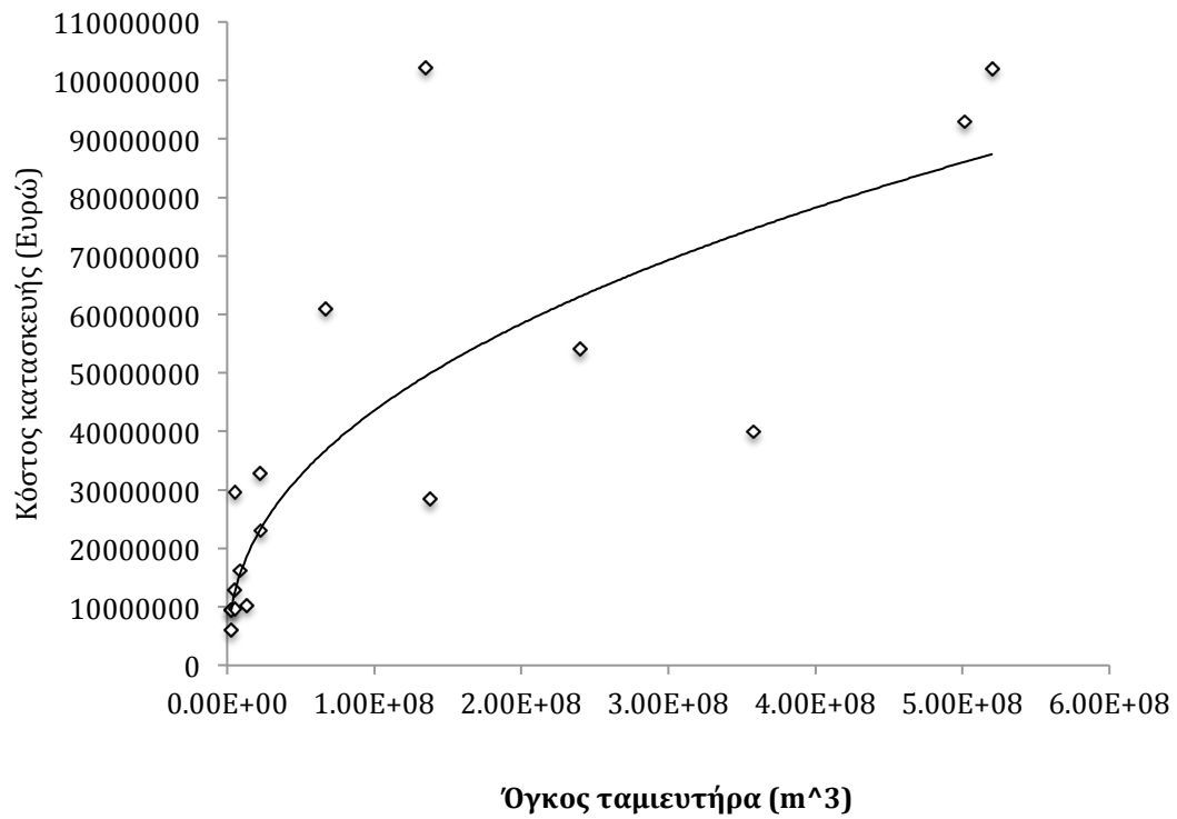
Σχήμα 8.3 Η συνεχής καμπύλη αντιστοιχεί στη \kappa_d = 18\,222 \cdot k^{0.42} . Με \blacklozenge συμβολίζεται η συσχέτιση \kappa_d - k των ταμιευτήρων που χρησιμοποιήθηκαν.
