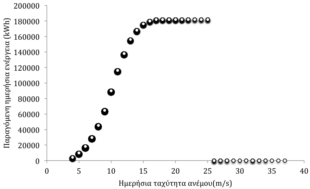
Σχήμα 6.2 Η ημερήσια παραγόμενη ενέργεια της ανεμογεννήτριας συναρτίζεται της ημερήσιας ταχύτητας ανέμου με χρήση των μέσων ημερήσιων ταχυτήτων ανέμου
