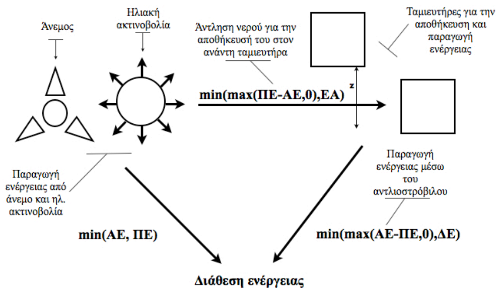
Σχήμα 3.1 Σκαρίφημα περιγραφής της λειτουργίας του συστήματος όπου ΑΕ είναι η απαιτούμενη ενέργεια δηλαδή η ενέργεια που ζητείται, ΠΕ είναι η παραγόμενη ενέργεια από τις αιολικές μηχανές και τα φωτοβολταϊκά, ΕΑ η ενέργεια που απαιτείται ώστε να αντληθεί όλη η διαθέσιμη ποσότητα νερού του κατάντη ταμιευτήρα, ΔΕ είναι η διαθέσιμη υδροηλεκτρική ενέργεια του ανάντη ταμιευτήρα.
