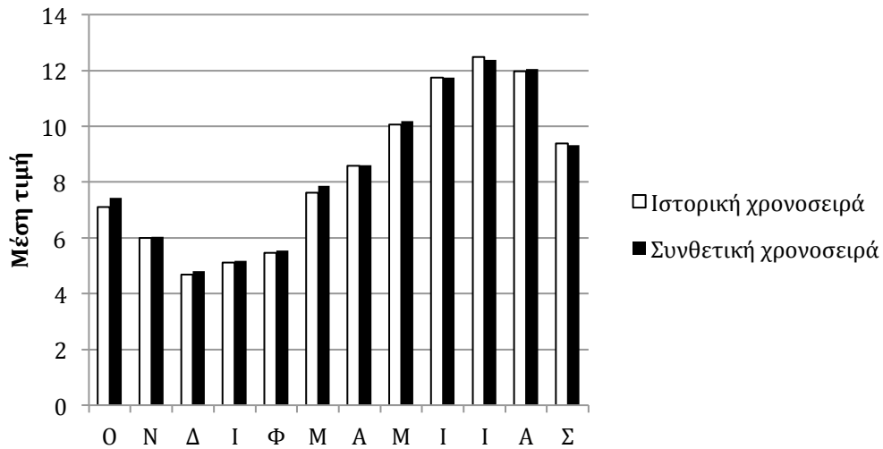
Σχήμα Β.5 Ραβδόγραμμα σύγκρισης των μέσων τιμών της διάρκειας ηλιοφάνειας σε μηνιαία κλίμακα για την ιστορική και συνθετική χρονοσειρά.
