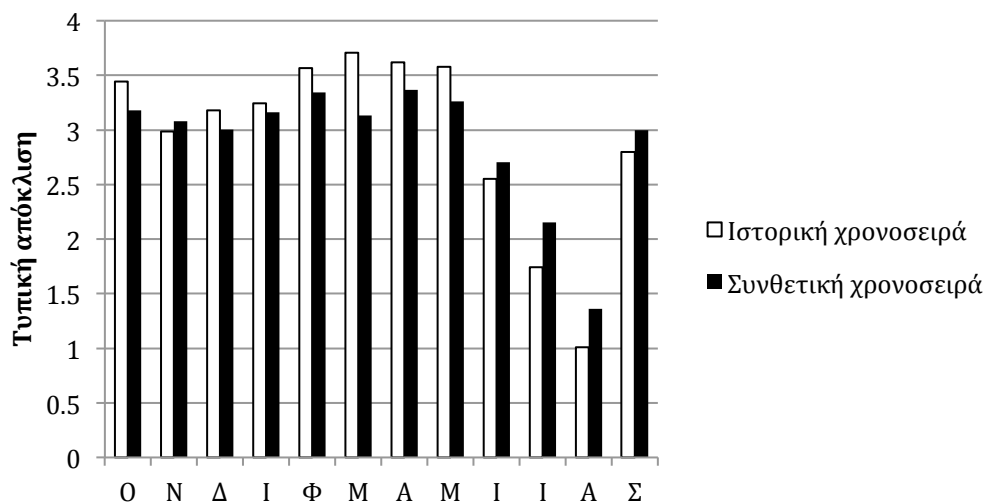
Σχήμα Β.2 Ραβδόγραμμα σύγκρισης των τυπικών αποκλίσεων της διάρκειας ηλιοφάνειας σε ημερήσια κλίμακα για την ιστορική και συνθετική χρονοσειρά.
