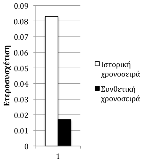
Σχήμα Β.27 Ραβδόγραμμα σύγκρισης του συντελεστή ετεροσυσχέτισης μηδενικής υστέρησης της διάρκειας ηλιοφάνειας και της ταχύτητας ανέμου για την ιστορική και συνθετική χρονοσειρά σε ετήσια κλίμακα.
