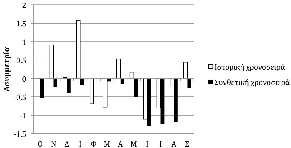
Σχήμα Α.7 Ραβδόγραμμα σύγκρισης των συντελεστών ασυμμετρίας της διάρκειας ηλιοφάνειας σε μηνιαία κλίμακα για την ιστορική και συνθετική χρονοσειρά.
