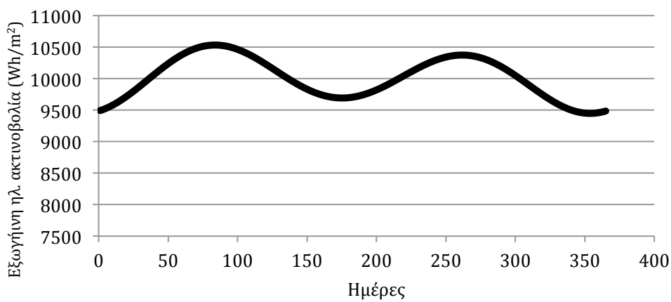
Σχήμα Δ.5 Ημερήσια εξωγήινη ηλιακή ακτινοβολία σε επίπεδο με κλίση 34°.
