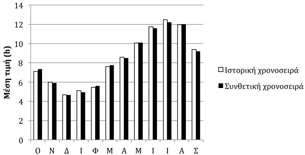
Σχήμα Α.5 Ραβδόγραμμα σύγκρισης των μέσων τιμών της διάρκειας ηλιοφάνειας σε μηνιαία κλίμακα για την ιστορική και συνθετική χρονοσειρά.
