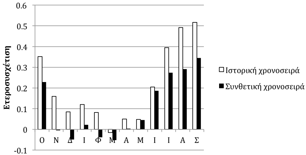
Σχήμα Β.25 Ραβδόγραμμα σύγκρισης των συντελεστών ετεροσυσχέτισης μηδενικής υστέρησης της διάρκειας ηλιοφάνειας και της ταχύτητας ανέμου για την ιστορική και συνθετική χρονοσειρά σε ημερήσια κλίμακα.
