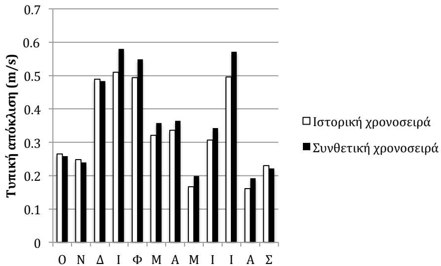
Σχήμα A.18 Ραβδόγραμμα σύγκρισης των τυπικών αποκλίσεων της ταχύτητας ανέμου σε μηνιαία κλίμακα για την ιστορική και συνθετική χρονοσειρά.
