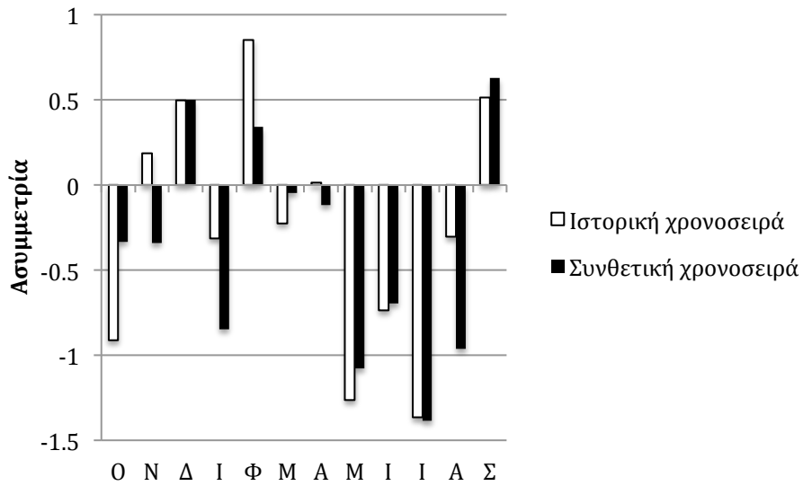
Σχήμα Β.19 Ραβδόγραμμα σύγκρισης των ασυμμετριών της ταχύτητας ανέμου σε μηνιαία κλίμακα για την ιστορική και συνθετική χρονοσειρά.
