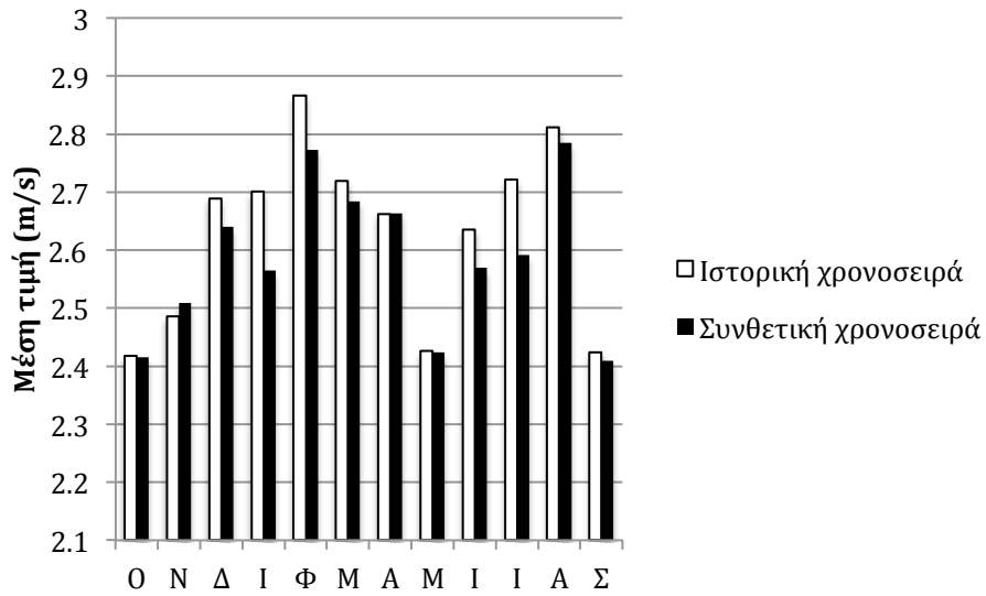
Σχήμα A.17 Ραβδόγραμμα σύγκρισης των μέσων τιμών της ταχύτητας ανέμου σε μηνιαία κλίμακα για την ιστορική και συνθετική χρονοσειρά.
