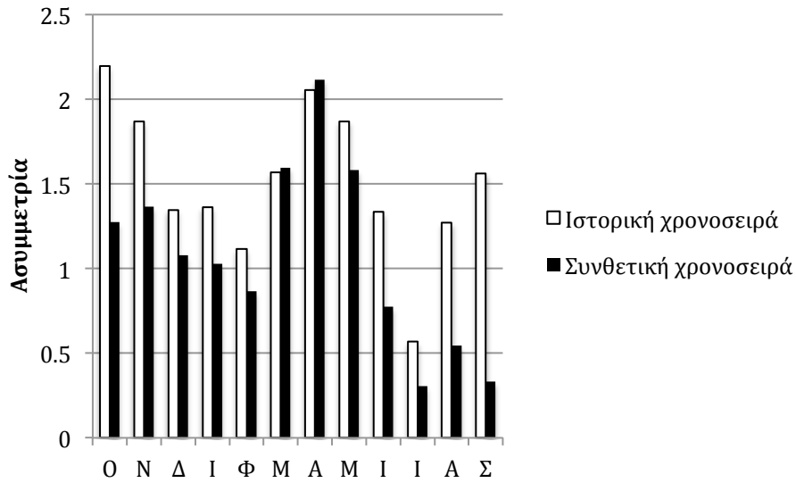
Σχήμα Β.15 Ραβδόγραμμα σύγκρισης των συντελεστών ασυμμετρίας της ταχύτητας ανέμου σε ημερήσια κλίμακα για την ιστορική και συνθετική χρονοσειρά.
