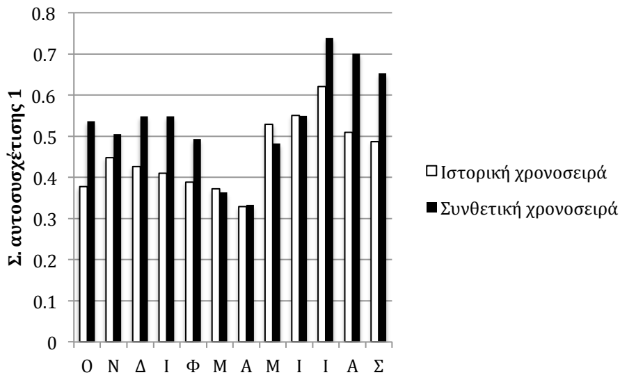
Σχήμα Β.16 Ραβδόγραμμα σύγκρισης των συντελεστών αυτοσυσχέτισης πρώτης τάξης της ταχύτητας ανέμου σε ημερήσια κλίμακα για την ιστορική και συνθετική χρονοσειρά.
