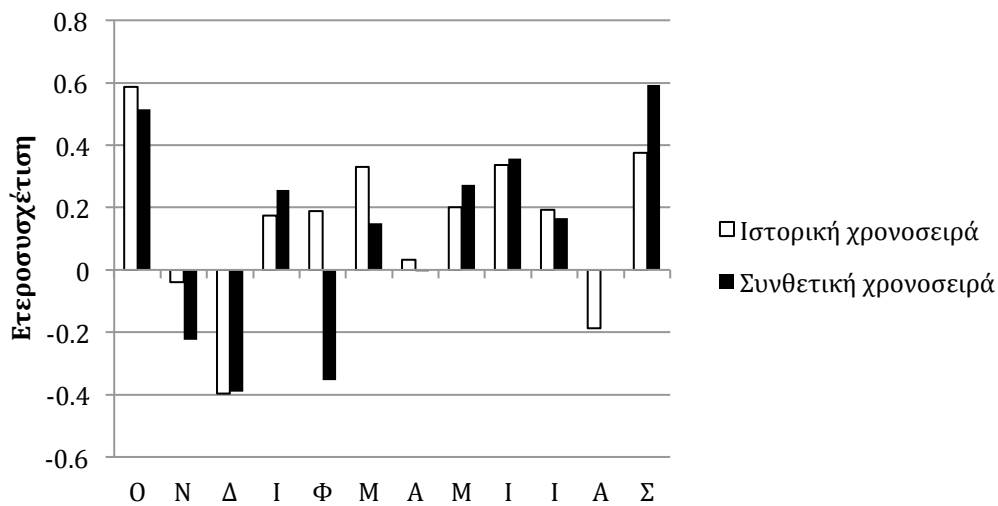
Σχήμα Β.26 Ραβδόγραμμα σύγκρισης των συντελεστών ετεροσυσχέτισης μηδενικής υστέρησης της διάρκειας ηλιοφάνειας και της ταχύτητας ανέμου για την ιστορική και συνθετική χρονοσειρά σε μηνιαία κλίμακα.
