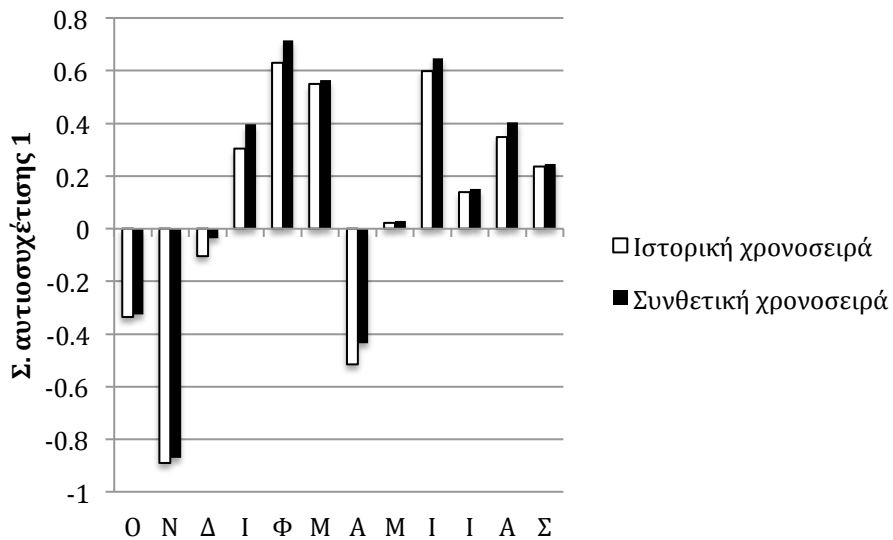
Σχήμα Β.20 Ραβδόγραμμα σύγκρισης των συντελεστών αυτοσυσχέτισης πρώτης τάξης της ταχύτητας ανέμου σε μηνιαία κλίμακα για την ιστορική και συνθετική χρονοσειρά.
