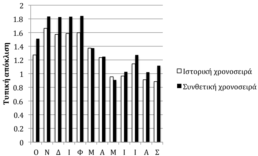
Σχήμα Β.14 Ραβδόγραμμα σύγκρισης των τυπικών αποκλίσεων της ταχύτητας ανέμου σε ημερήσια κλίμακα για την ιστορική και συνθετική χρονοσειρά.
