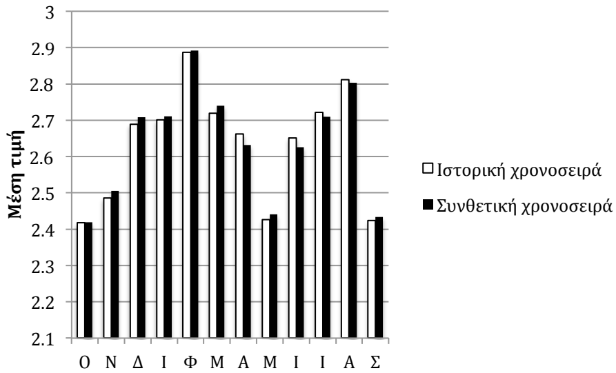
Σχήμα Β.13 Ραβδόγραμμα σύγκρισης των μέσων τιμών της ταχύτητας ανέμου σε ημερήσια κλίμακα για την ιστορική και συνθετική χρονοσειρά.
