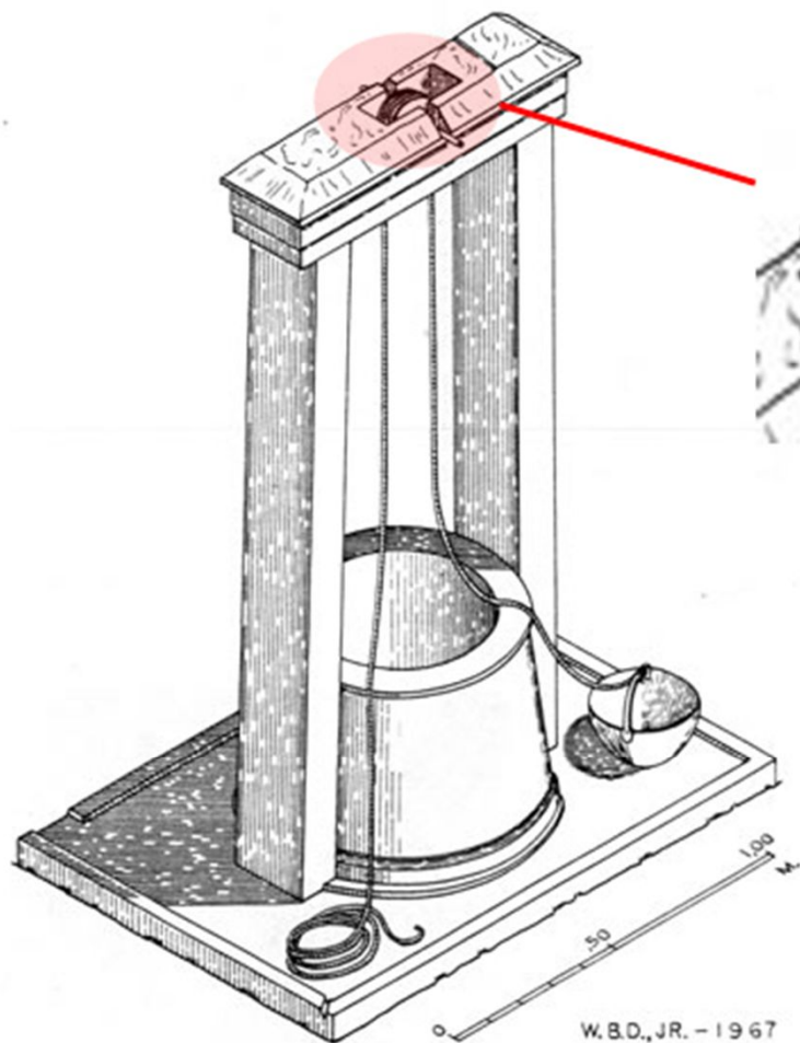
Αναπαράσταση της λειτουργίας του μηχανισμού άντλησης του Φρέατος Α660 από την Αγορά της Αθήνας πηγή: http://www.ascsa.net
