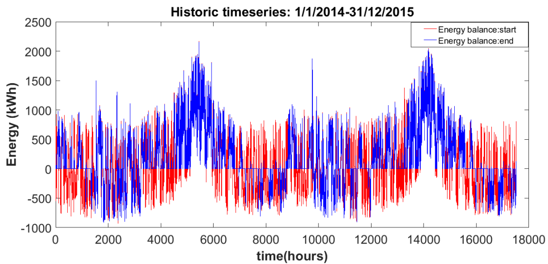
Διάγραμμα 4-22: Αρχικό και τελικό ισοζύγιο όπως διαμορφώνεται μετά την αναρρύθμιση μέσω της αντλησιοταμίευσης
