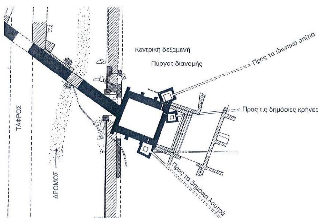
Εικόνα 13. Η κεντρική δεξαμενή με τα τρία φρεάτια που λειτουργούσαν ως πύργοι διανομής νερού στην πόλη. Πηγή: Καραδέδος, 2000, σελ.60
