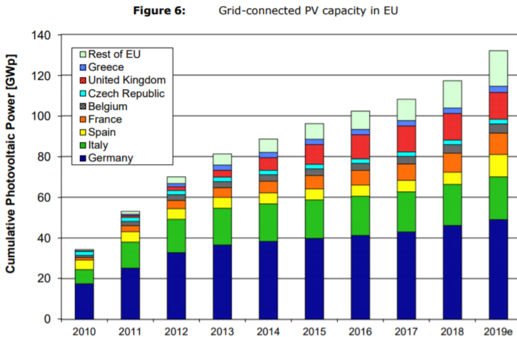
Διάγραμμα 2: Αθροιστική ισχύς συνδεδεμένων στο δίκτυο φωτοβολταϊκών στην Ευρώπη. Πηγή: PV Status Report 2019 [44]
