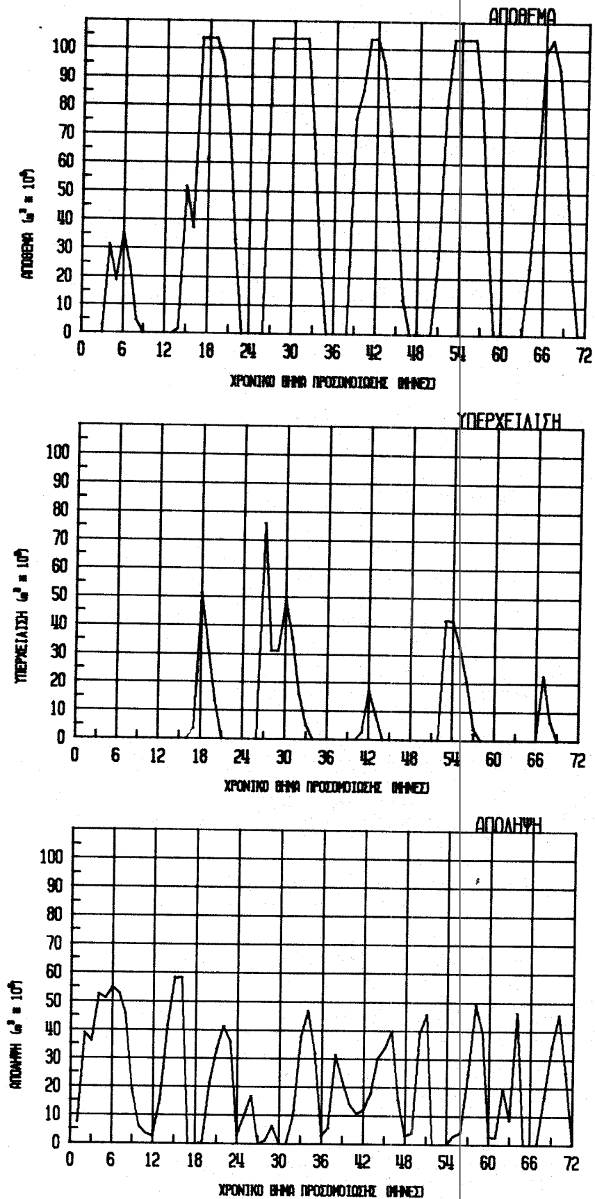
Σχ. 1 Λειτουργικά μεγέθη ταμειυτήρα Ευήνου από προσομύωση του συστήματος Μόρνου-Ευήνου με βάση τα ιστορικά δεδομένα της περιόδου 1979-80 έως 1984-85
