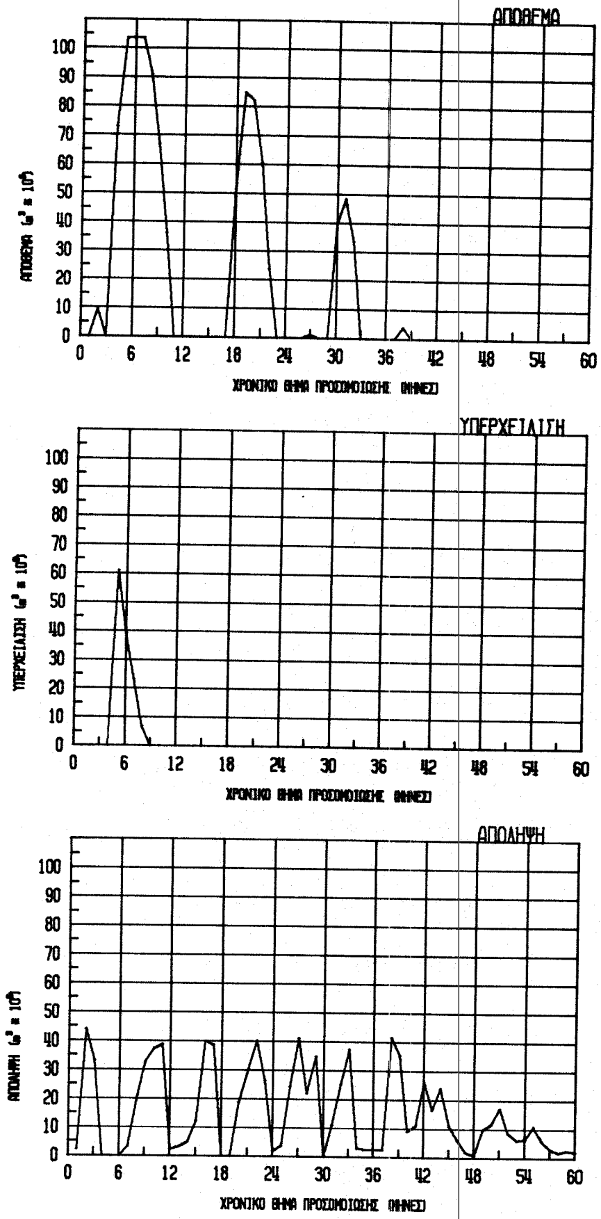
Σχ. 2 Λειτουργικά μεγέθη ταμειυτήρα Εύηνου από προσομύωση του συστήματος Μόρνου-Εύηνου με βάση τα ιστορικά δεδομένα της περιόδου 1985-86 έως 1989-90
