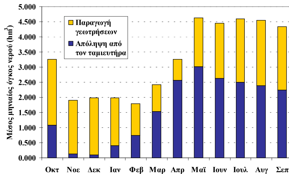
Σχήμα Β6: Μέση μηνιαία απόληψη από τον ταμιευτήρα Αποσελέμη και τις γεωτρήσεις.
