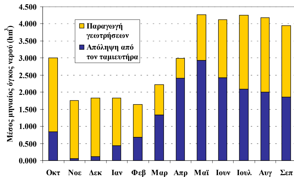
Σχήμα Β20: Μέση μηνιαία απόληψη από τον ταμιευτήρα Αποσελέμη και τις γεωτρήσεις.
