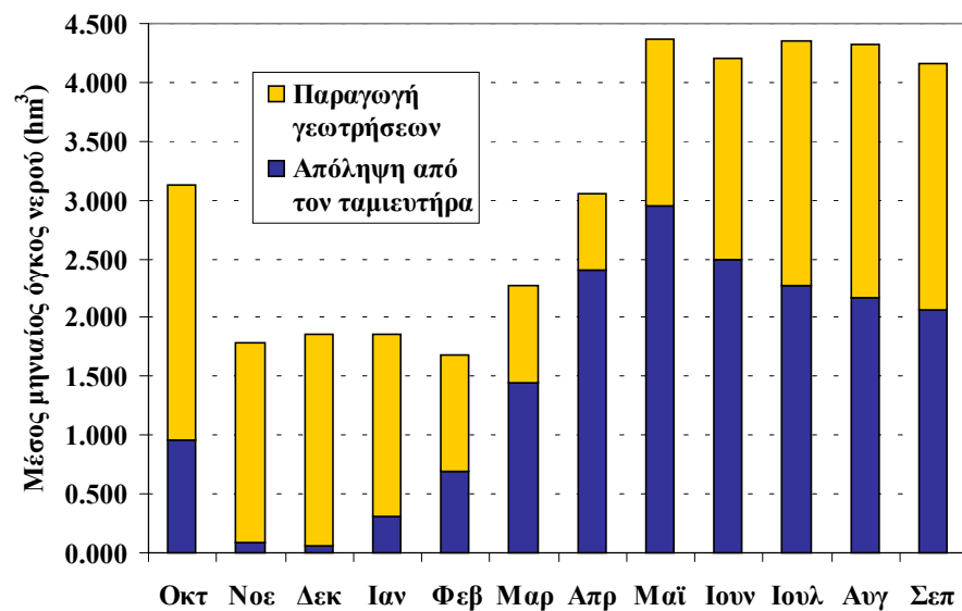
Σχήμα Β10: Μέση μηνιαία απόληψη από τον ταμιευτήρα Αποσελέμη και τις γεωτρήσεις.
