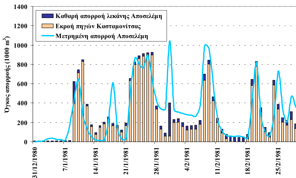
Σχήμα 3.11: Απεικόνιση προσομοιωμένου και δειγματικού υδρογραφήματος για την περίοδο 31/12/80 μέχρι 1/3/81.
