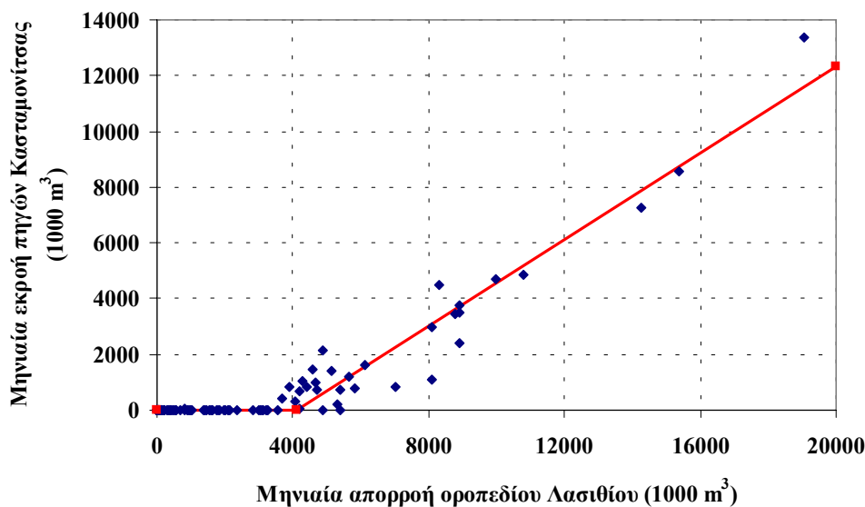
Σχήμα 3.12: Συσχέτιση εκροής πηγών Κασταμονίτσας – απορροής Οροπεδίου Λασιθίου (Σενάριο 1, 30% επικοινωνία).
