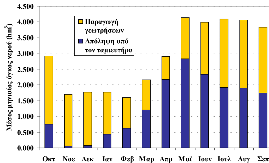
Σχήμα Β19: Μέση μηνιαία απόληψη από τον ταμιευτήρα Αποσελέμη και τις γεωτρήσεις.
