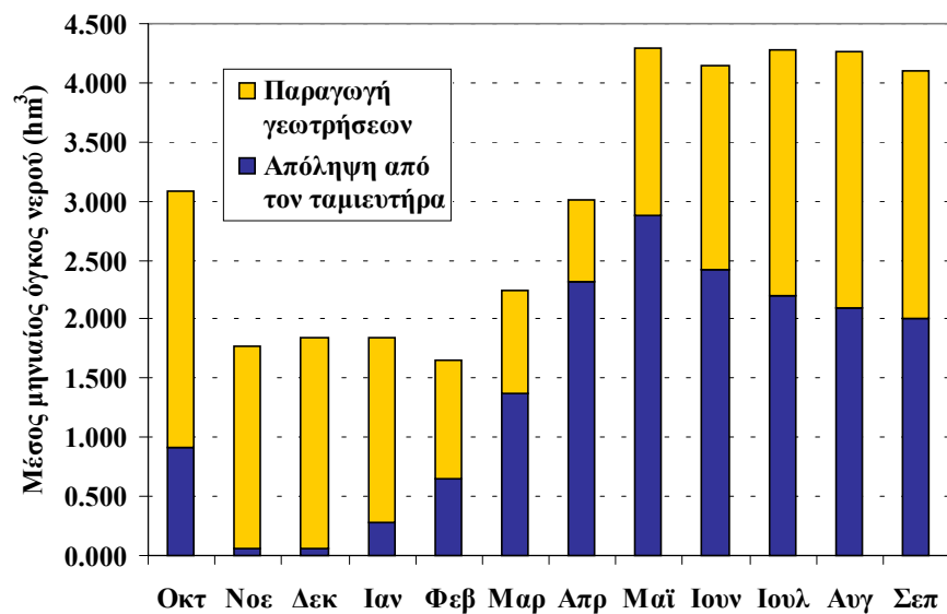
Σχήμα Β16: Μέση μηνιαία απόληψη από τον ταμιευτήρα Αποσελέμη και τις γεωτρήσεις.
