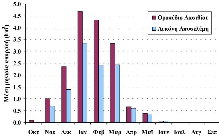
Σχήμα 4.3: Μέση μηνιαία απορροή λεκάνης Αποσελέμη και Οροπεδίου Λασιθίου.
