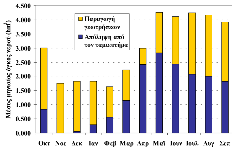
Σχήμα Β22: Μέση μηνιαία απόληψη από τον ταμιευτήρα Αποσελέμη και τις γεωτρήσεις.
