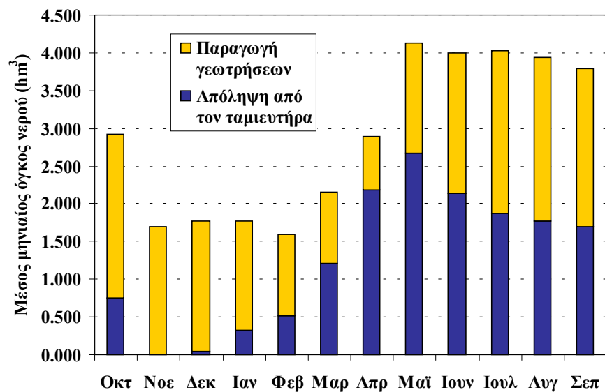
Σχήμα Β23: Μέση μηνιαία απόληψη από τον ταμιευτήρα Αποσελέμη και τις γεωτρήσεις.
