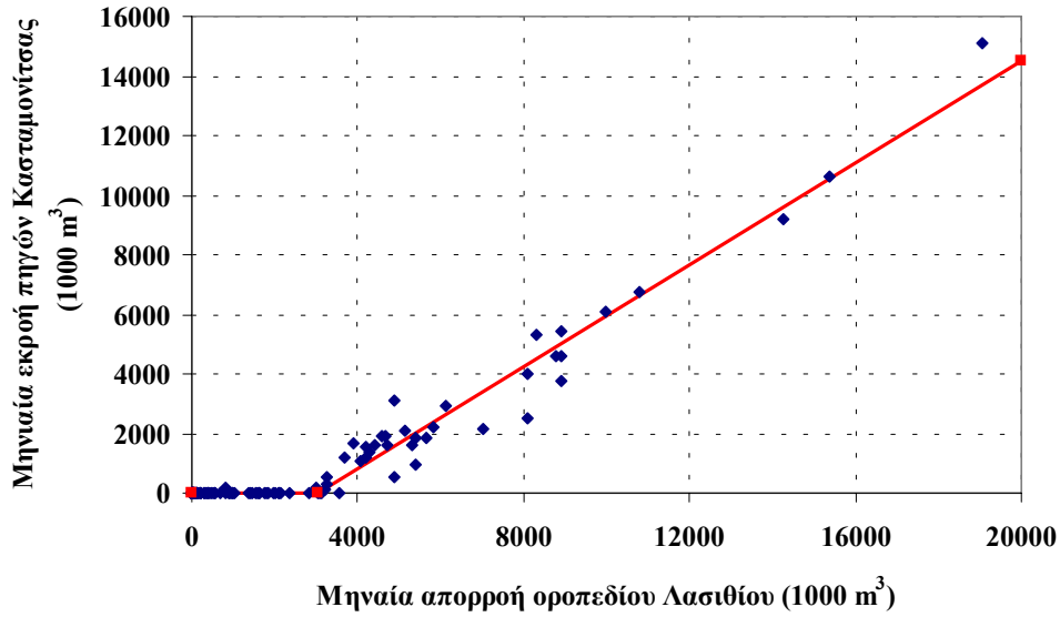
Σχήμα 3.13: Συσχέτιση εκροής πηγών Κασταμονίτσας – απορροής Οροπεδίου Λασιθίου (Σενάριο 2, 50% επικοινωνία).
