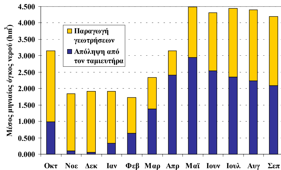
Σχήμα Β5: Μέση μηνιαία απόληψη από τον ταμιευτήρα Αποσελέμη και τις γεωτρήσεις.
