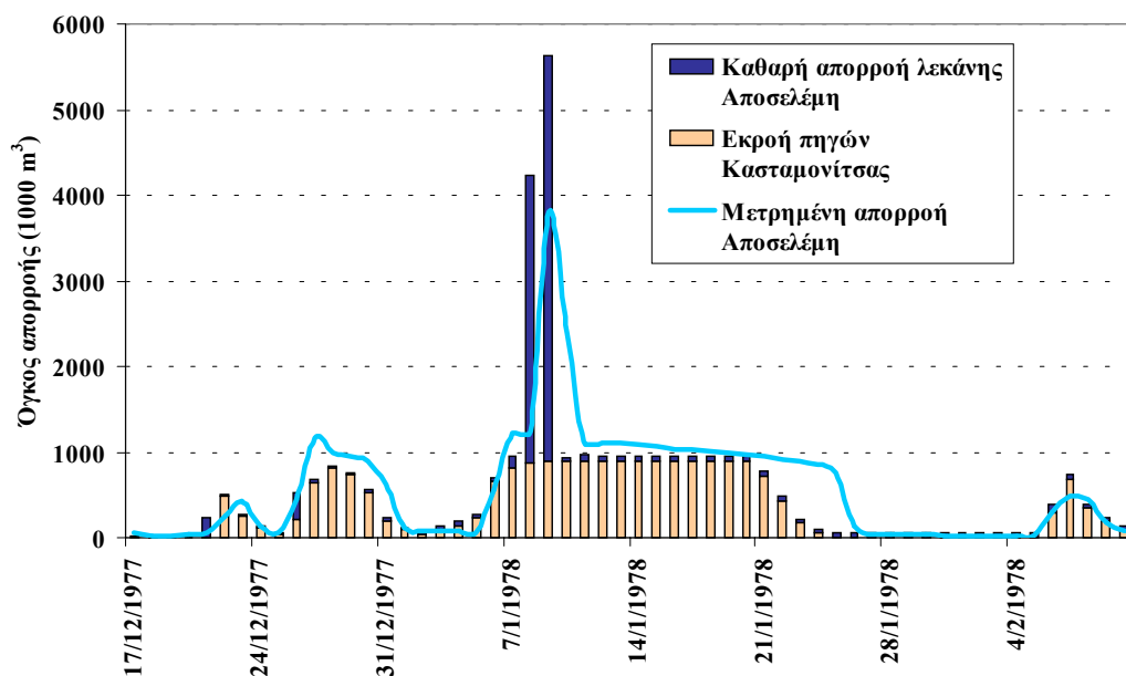
Σχήμα 3.10: Απεικόνιση προσομοιωμένου και δειγματικού υδρογραφήματος για την περίοδο 17/12/77 μέχρι 10/2/78.
