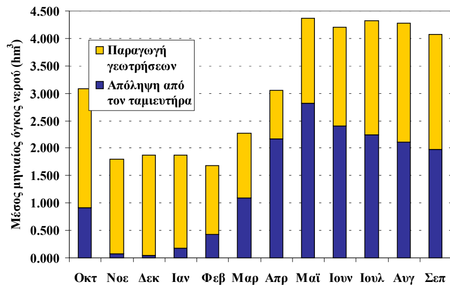
Σχήμα Β17: Μέση μηνιαία απόληψη από τον ταμιευτήρα Αποσελέμη και τις γεωτρήσεις.
