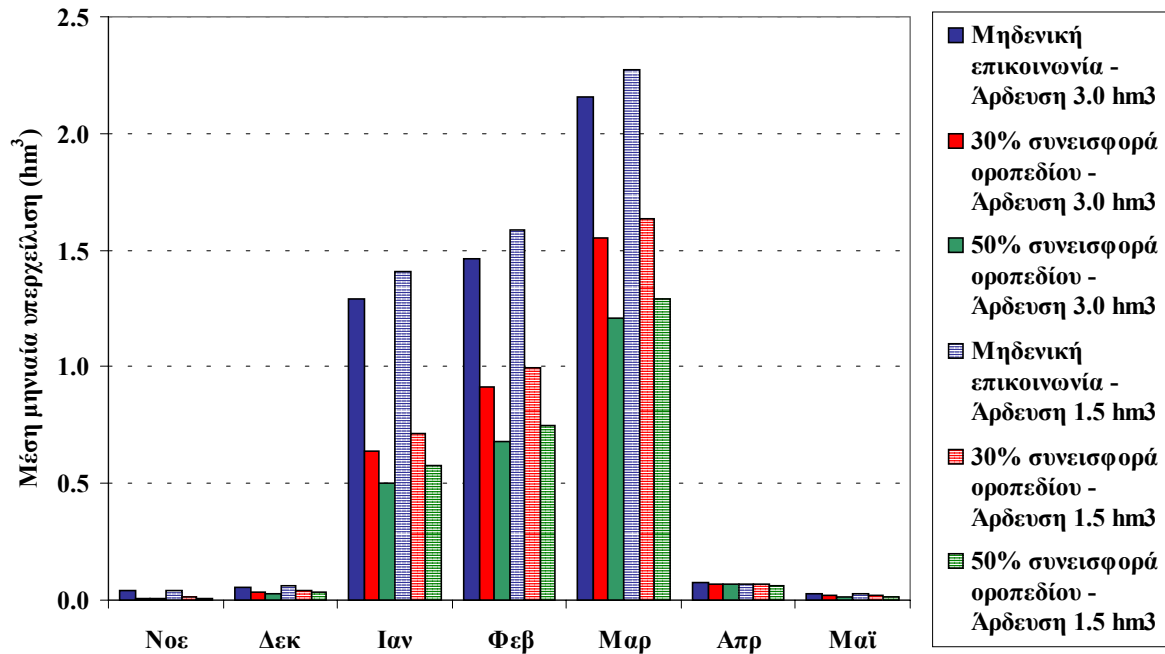
Σχήμα 4.11: Μέσες μηνιαίες υπερχειλίσεις ταμιευτήρα Αποσελέμη για τα τρία ποσοστά επικοινωνίας των λεκανών Οροπεδίου Λασιθίου και Αποσελέμη και τις δύο τιμές αρδευτικής απόληψης, για επίπεδο αξιοπιστίας του υδροσυστήματος ίσο με 95%.
