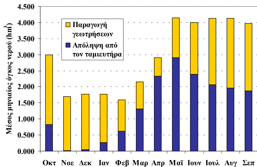
Σχήμα Β14: Μέση μηνιαία απόληψη από τον ταμιευτήρα Αποσελέμη και τις γεωτρήσεις.
