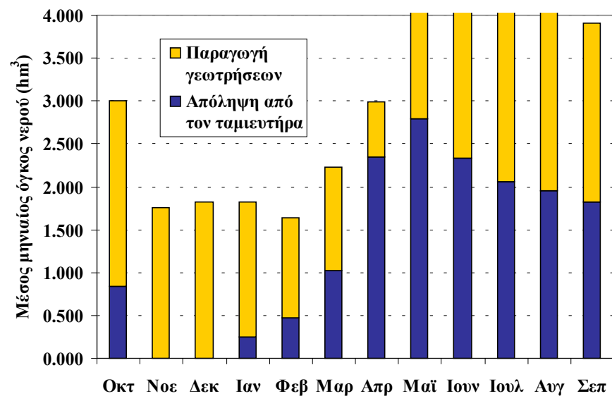
Σχήμα Β24: Μέση μηνιαία απόληψη από τον ταμιευτήρα Αποσελέμη και τις γεωτρήσεις.
