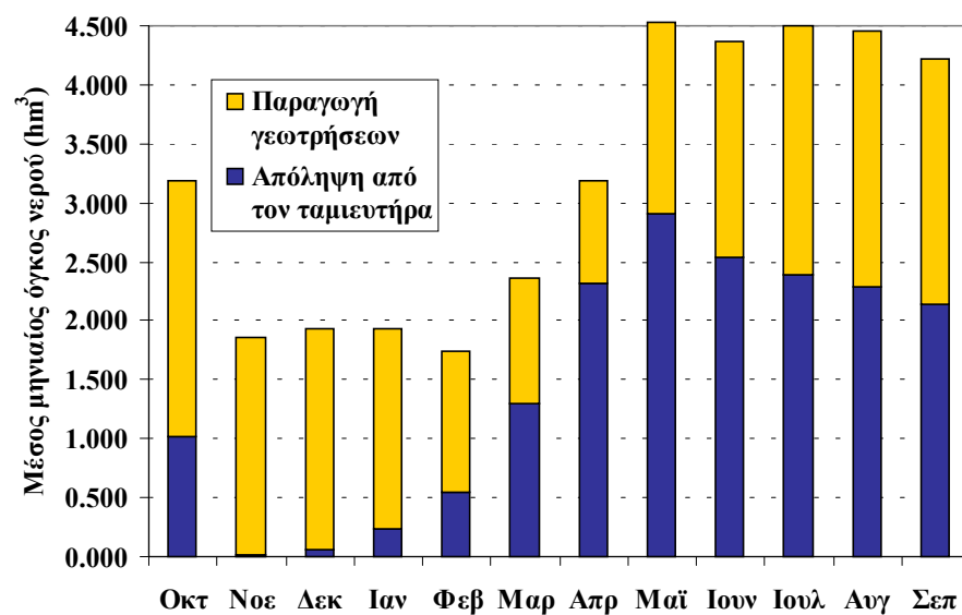
Σχήμα Β18: Μέση μηνιαία απόληψη από τον ταμιευτήρα Αποσελέμη και τις γεωτρήσεις.
