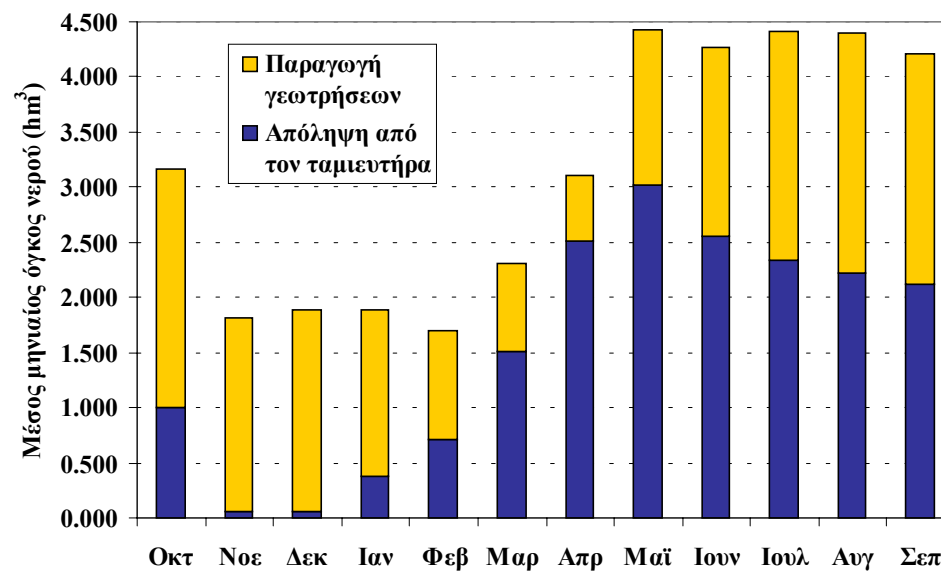
Σχήμα Β4: Μέση μηνιαία απόληψη από τον ταμιευτήρα Αποσελέμη και τις γεωτρήσεις.
