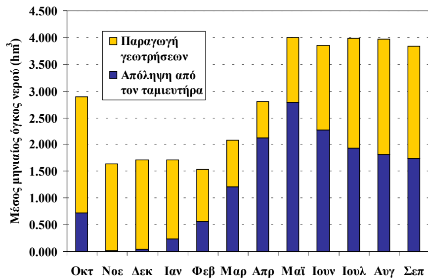
Σχήμα Β13: Μέση μηνιαία απόληψη από τον ταμιευτήρα Αποσελέμη και τις γεωτρήσεις.
