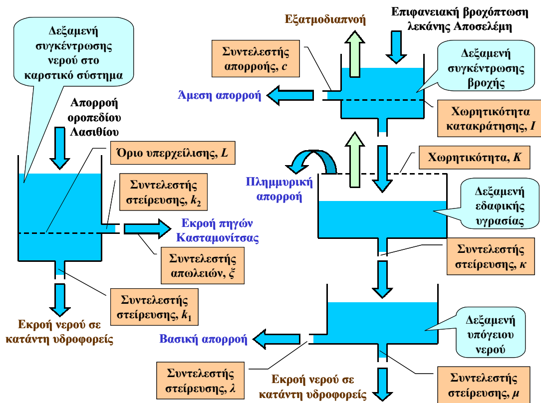
Σχήμα 3.5: Σχηματική απεικόνιση των συνιστωσών του μοντέλου υδατικού ισοζυγίου
